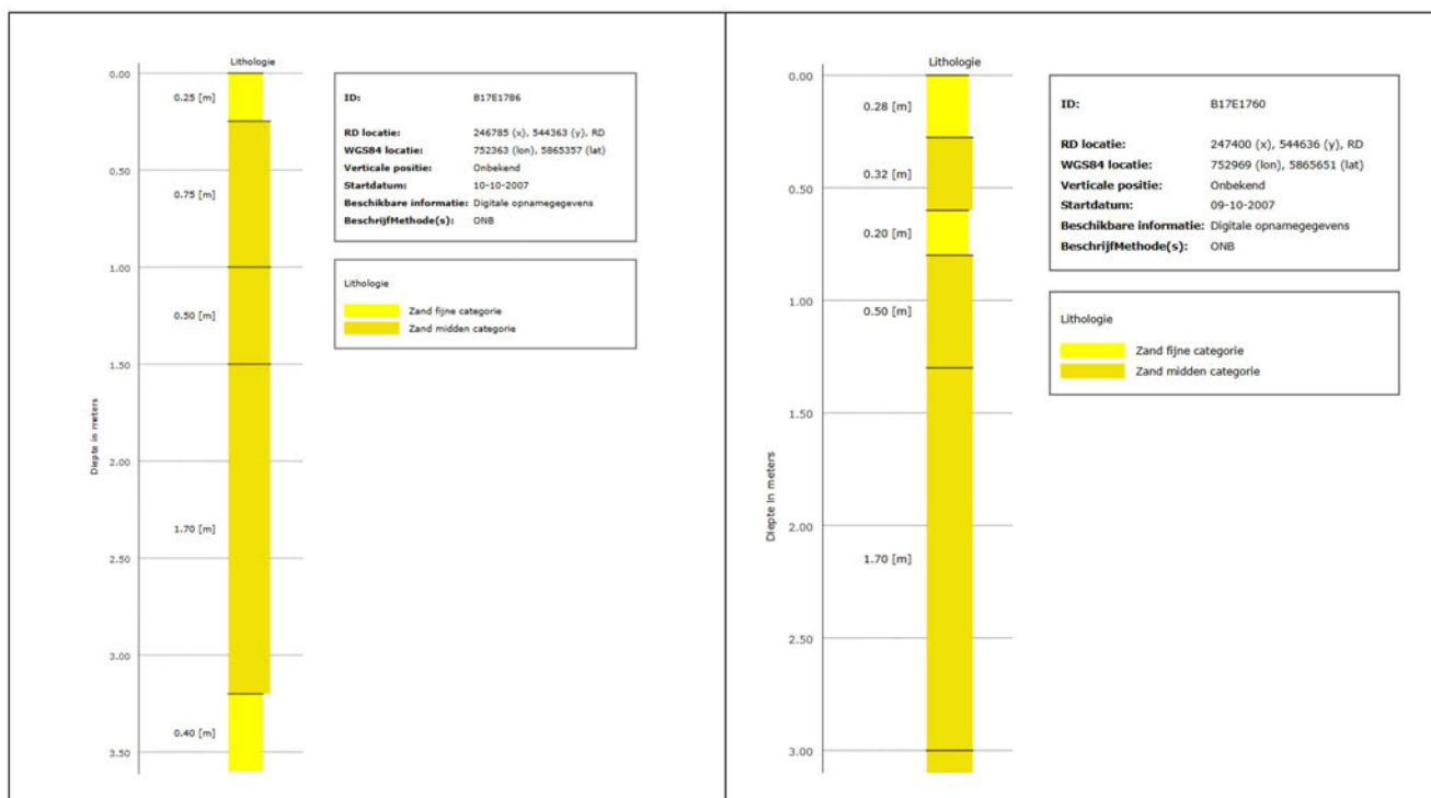
Figuur 6-1- Grondboringen 6 kruising westzijde (links) en oostzijde (rechts)
