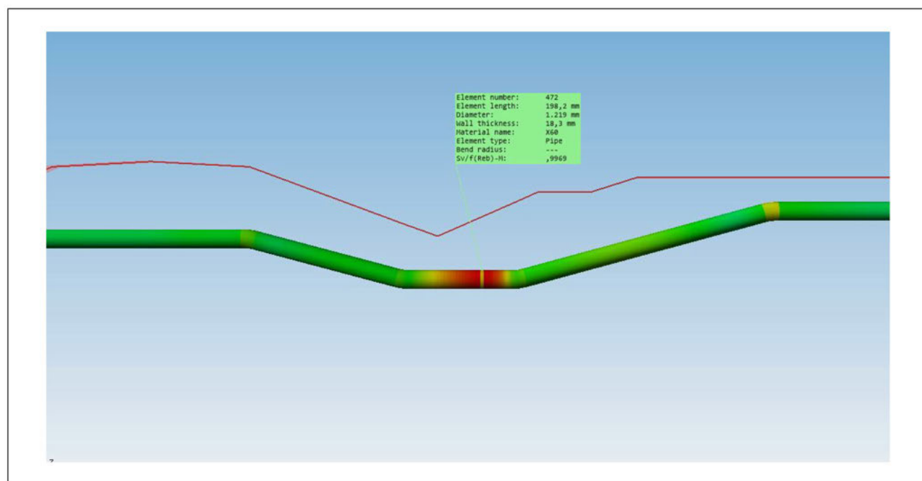
Figuur 6-4: Locatie van maximaal berekende spanning
