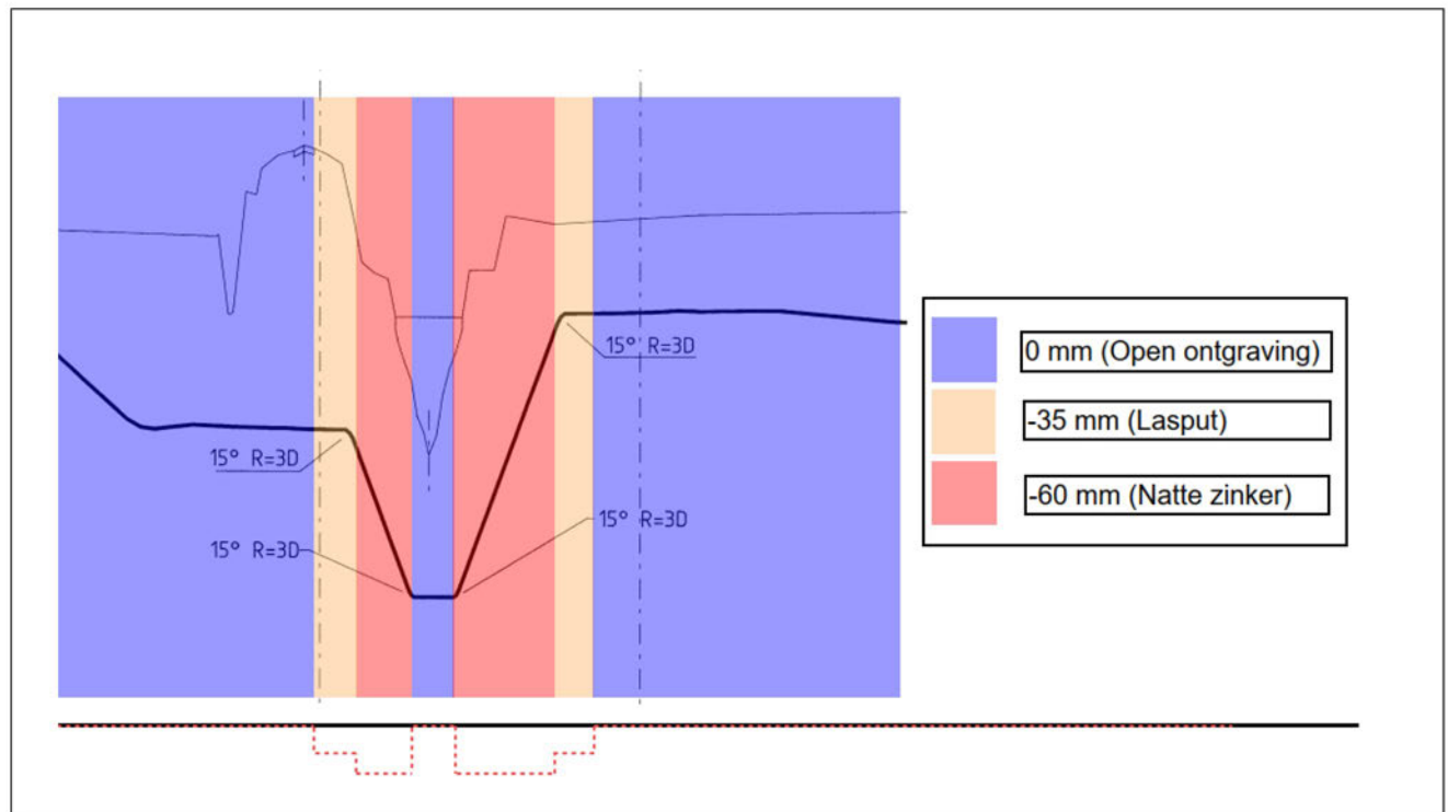
Figuur 6-3: Uitvoeringszakkingsverschil en schematische weergave bouwput
