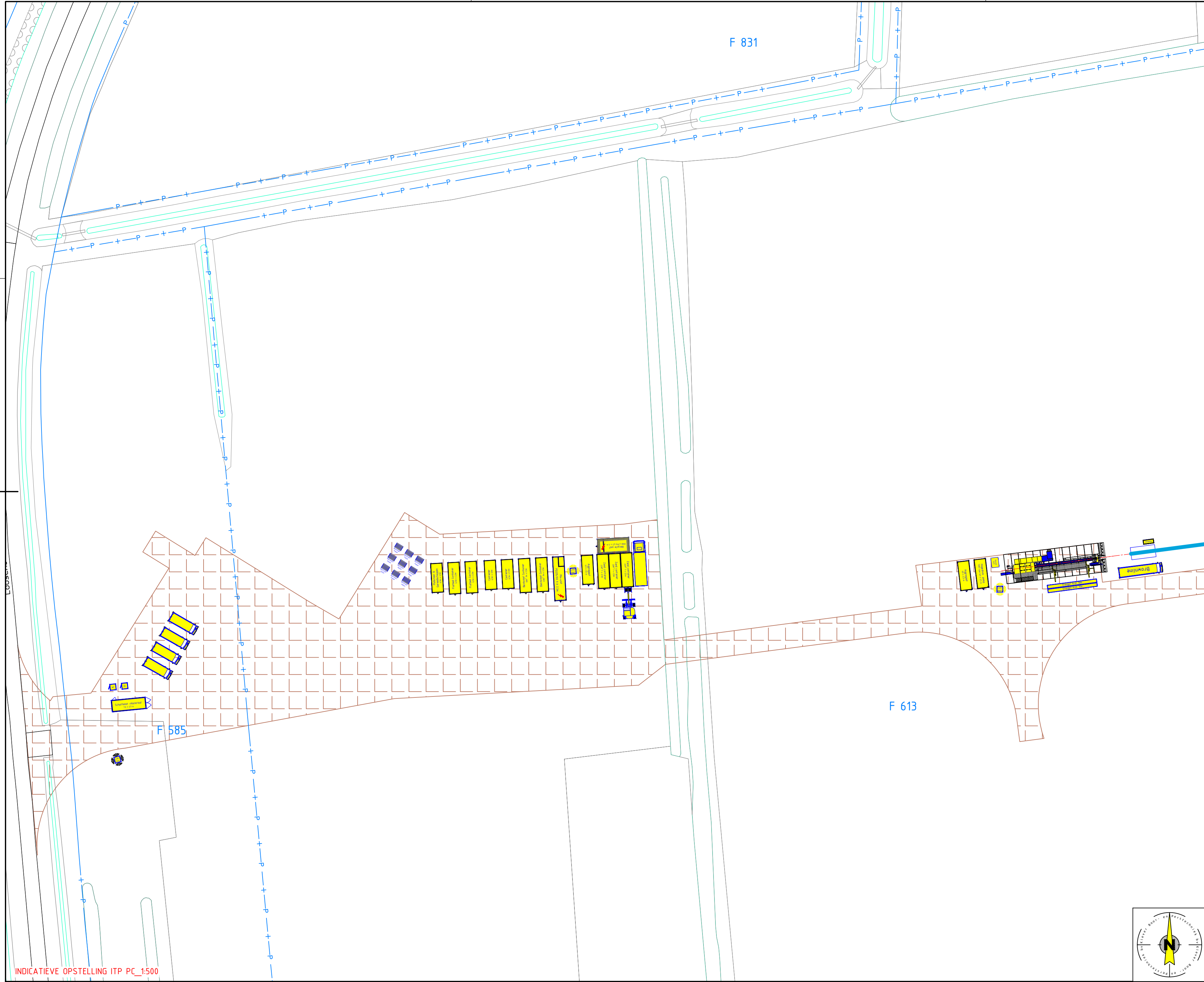
INDICATIEVE OPSTELLING ITP PC_1500
