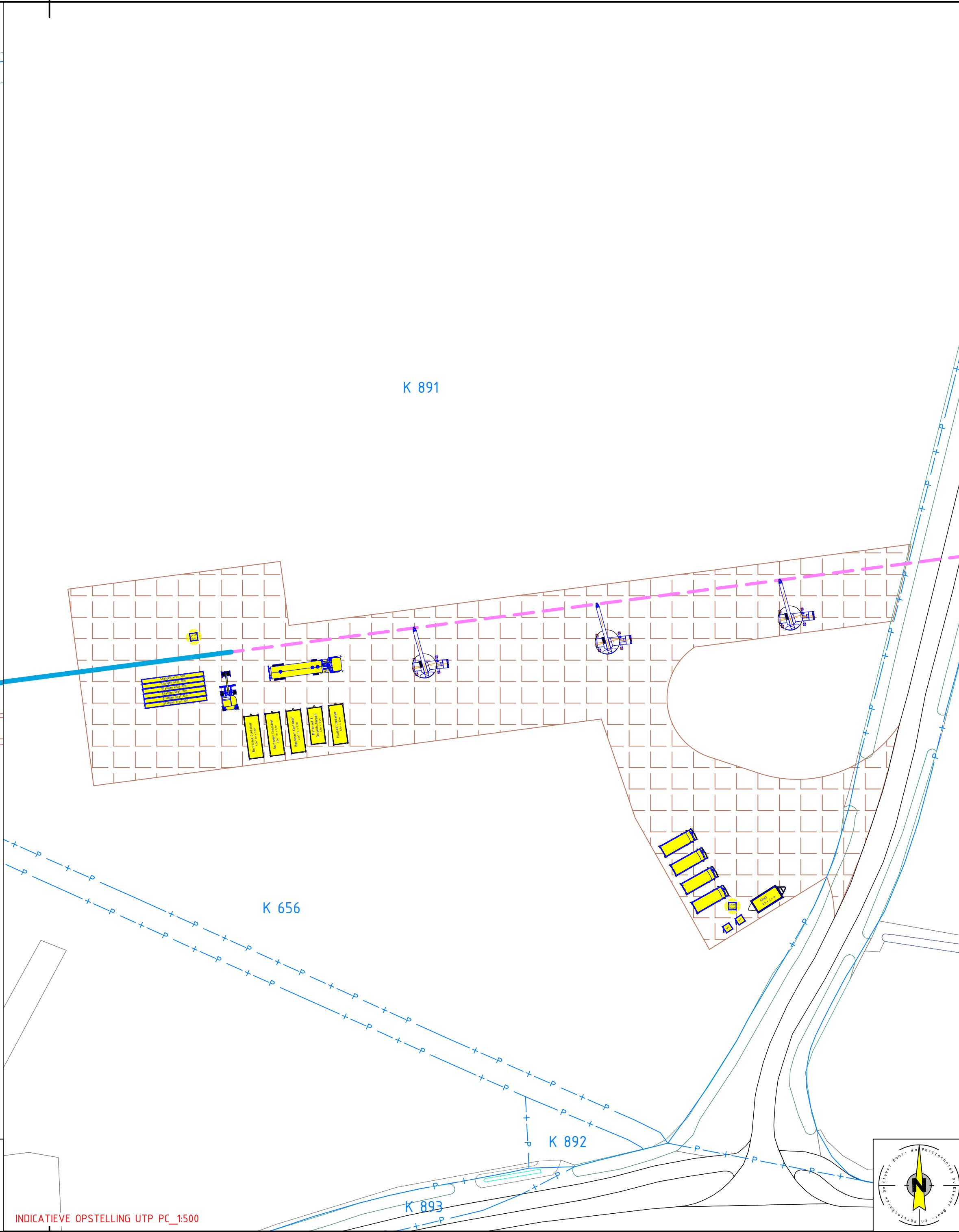
INDICATIEVE OPSTELLING UTP PC_1500
