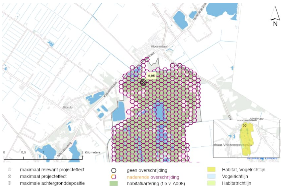
Figuur 11.5: De locatie in het Natura 2000-gebied Engbertsdijkswenen met de maximale relevante toename van stikstofdepositie op het leefgebied van Geoorde fuut (A008).
