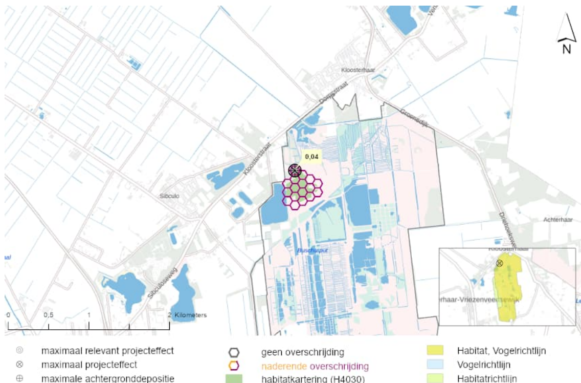
Figuur 11.2: De locatie in het Natura 2000-gebied Engbertsdijksvenen met de maximale relevante toename van stikstofdepositie op Droge heiden (H4030).
