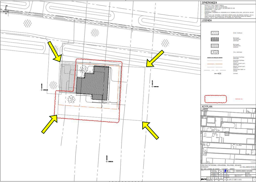
Figuur 3. Toekomstige situatie S-222, waarbij het hekwerk verkleind is ten opzicht van de huidige situatie (bron: N.V. Nederlandse Gasunie). De hoeken van het huidige hekwerk zijn zowel en in de huidige als in de toekomstige situatie gemarkeerd middels gele pijlen ter verduidelijking.
