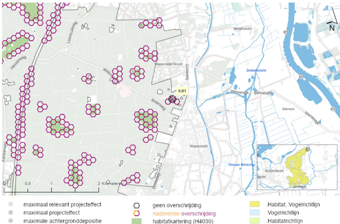
Figuur 25.5: De locatie in het Natura 2000-gebied Veluwe met de maximale relevante toename van stikstofdepositie op Drogen heiden (H4030).
