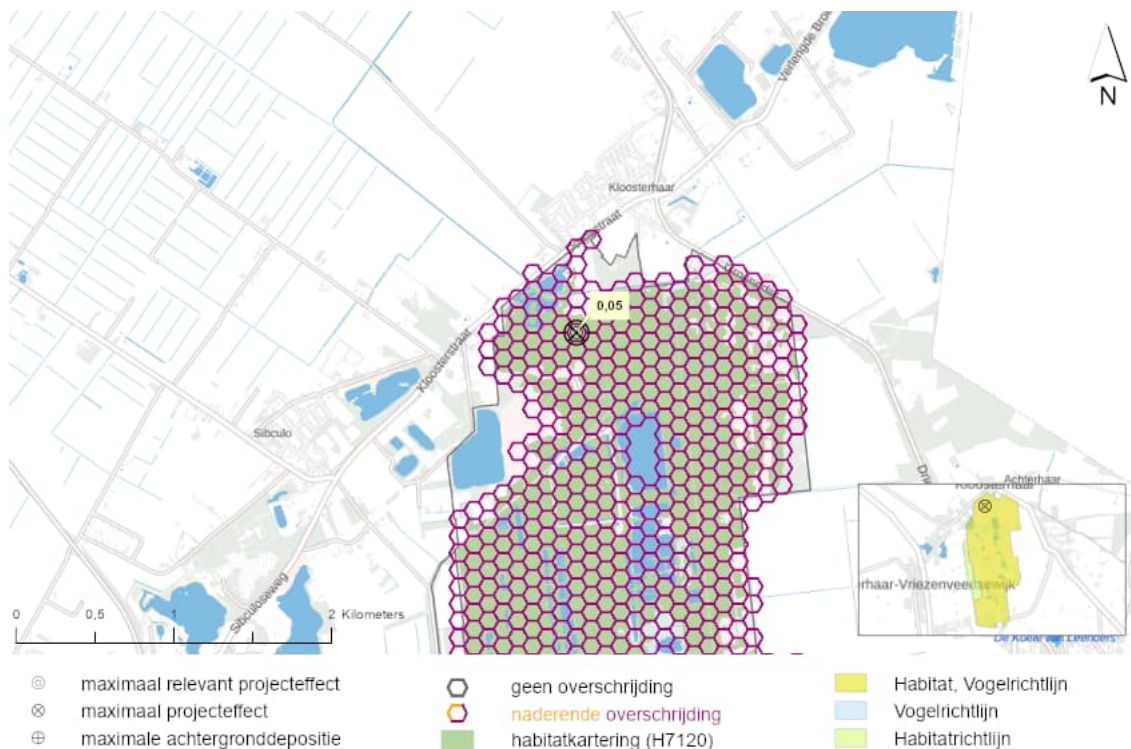
Figuur 11.4: De locatie in het Natura 2000-gebied Engbertsdijksvenen met de maximale relevante toename van stikstofdepositie op Herstellende hoogvenen (H7120).
