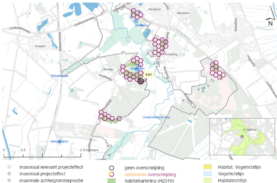
Figuur 14.2: De locatie in het Natura 2000-gebied Drentsche Aa-gebied met de maximale relevante toename van stikstofdepositie op Stuifzandheiden met struikhei (H2310).
