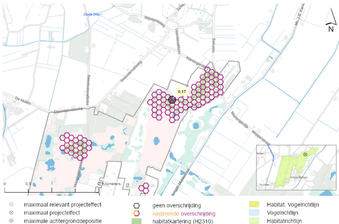
Figuur 4.2: De locatie in het Natura 2000-gebied Mantingerzand met de maximale relevante toename van stikstofdepositie op Stuifzandheiden met struikheide (H2310).
