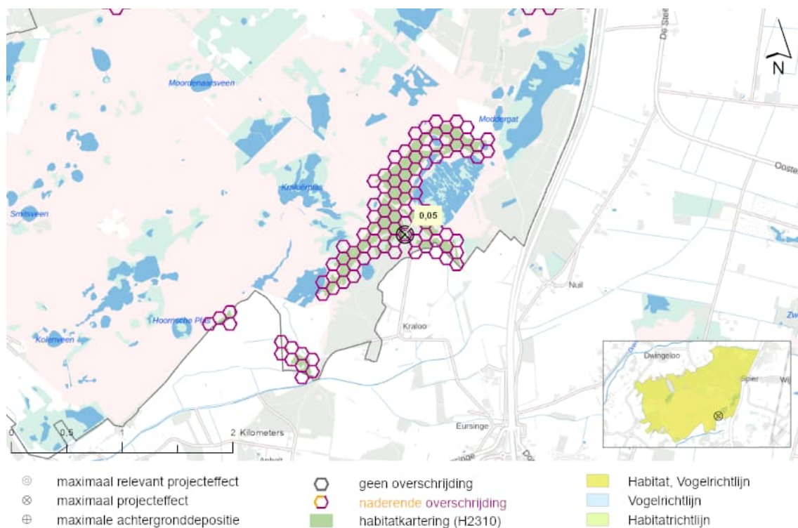
Figuur 10.2: De locatie in het Natura 2000-gebied Dwingelderveld met de maximale relevante toename van stikstofdepositie op Stuifzandheiden met struikhei (H2310).
