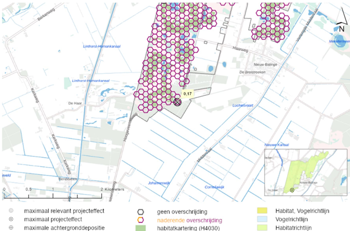
Figuur 4.8: De locatie in het Natura 2000-gebied Mantingerzand met de maximale relevante toename van stikstofdepositie op Droge heiden (H4030).
