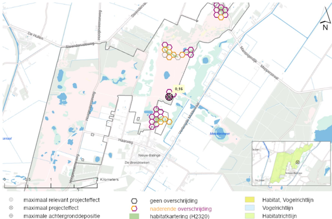
Figuur 4.3: De locatie in het Natura 2000-gebied Mantingerzand met de maximale relevante toename van stikstofdepositie op Binnenlandse kraaiheibegroeiingen (H2320).
