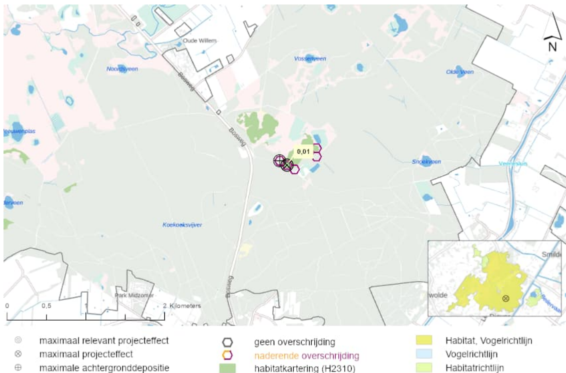
Figuur 13.2: De locatie in het Natura 2000-gebied Drents-Friese Wold & Leggelderveld met de maximale relevante toename van stikstofdepositie op Stufzandheiden met struikheide (H2310).
