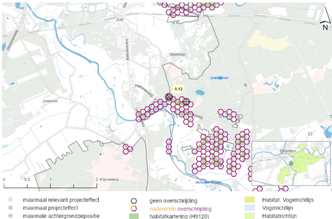
Figuur 6.16: De locatie in het Natura 2000-gebied Vecht- en Beneden-Reggegebied met de maximale relevante toename van stikstofdepositie op Beuken-eikenbossen met hultst (H9120).
