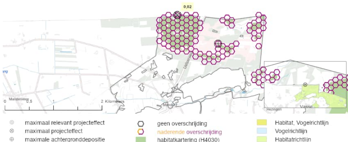
Figuur 17.3: De locatie in het Natura 2000-gebied Springendal & Dal van de Mosbeek met de maximale relevante toename van stikstofdepositie op Droge heiden (H4030).
