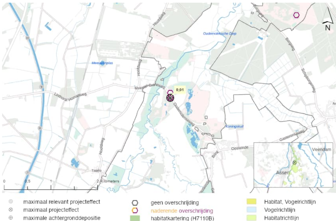
Figuur 14.11: De locatie in het Natura 2000-gebied Drentsche Aa-gebied met de maximale relevante toename van stikstofdepositie op Actieve hoogvenen (heideveentjes) (H7110B).
