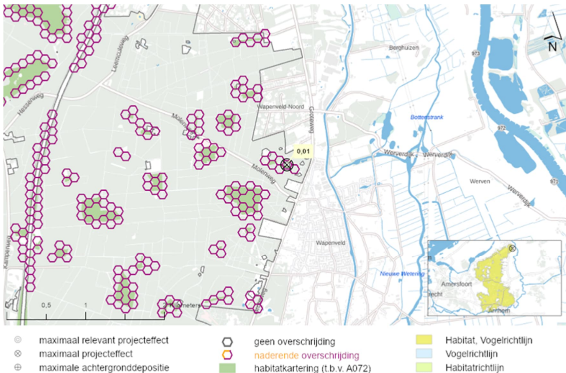
Figuur 25.10: De locatie in het Natura 2000-gebied Veluwe met de maximale relevante toename van stikstofdepositie op het leefgebied van Wespendif (A072).
