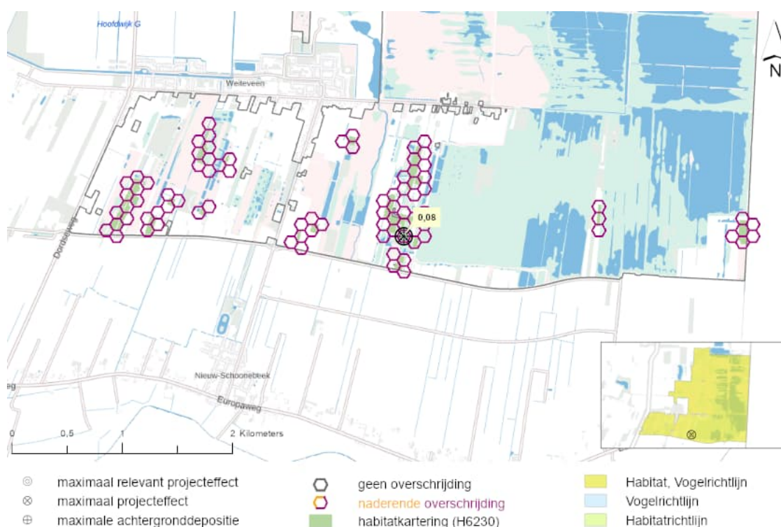
Figuur 8.2: De locatie in het Natura 2000-gebied Bargerveen met de maximale relevante toename van stikstofdepositie op Heischrale graslanden (H6230).
