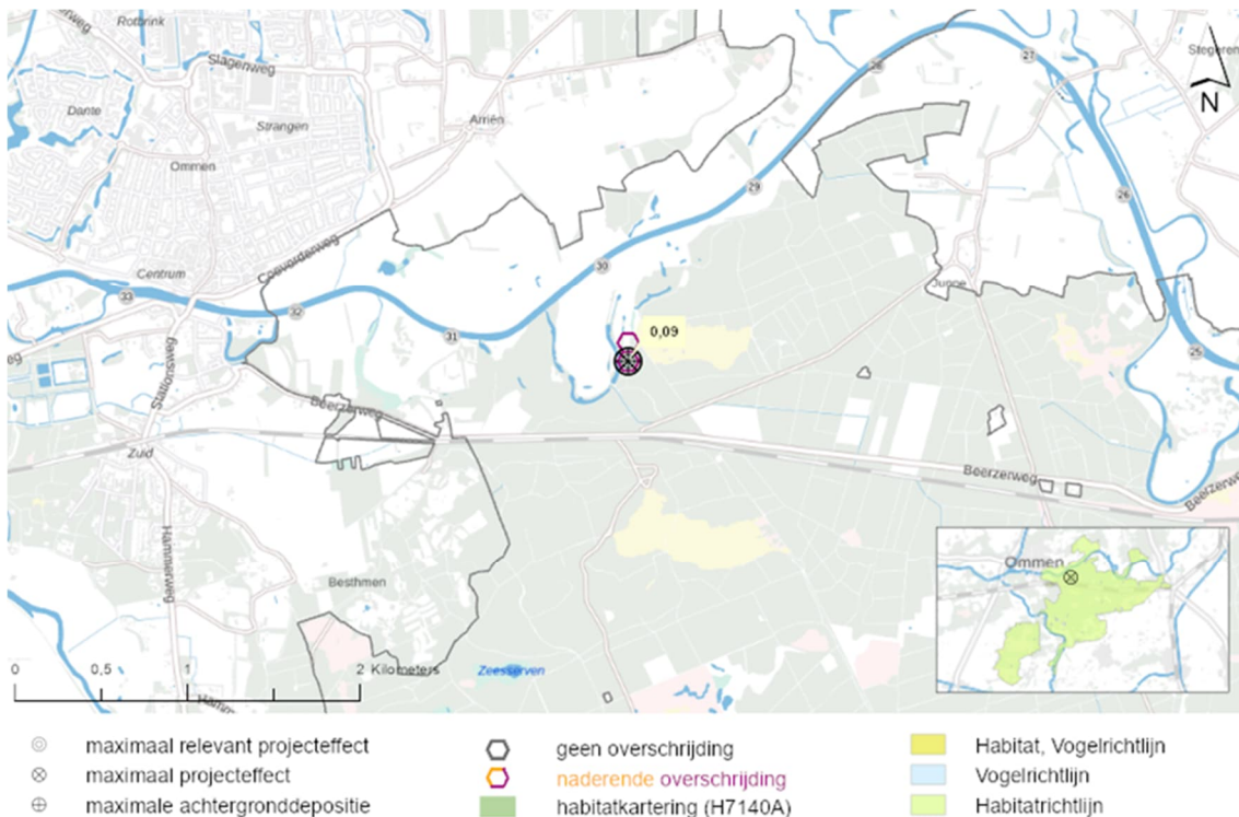
Figuur 6.14: De locatie in het Natura 2000-gebied Vecht- en Beneden-Reggegebied met de maximale relevante toename van stikstofdepositie op Overgangs- en trilvenen (trilvenen) (H7140A).
