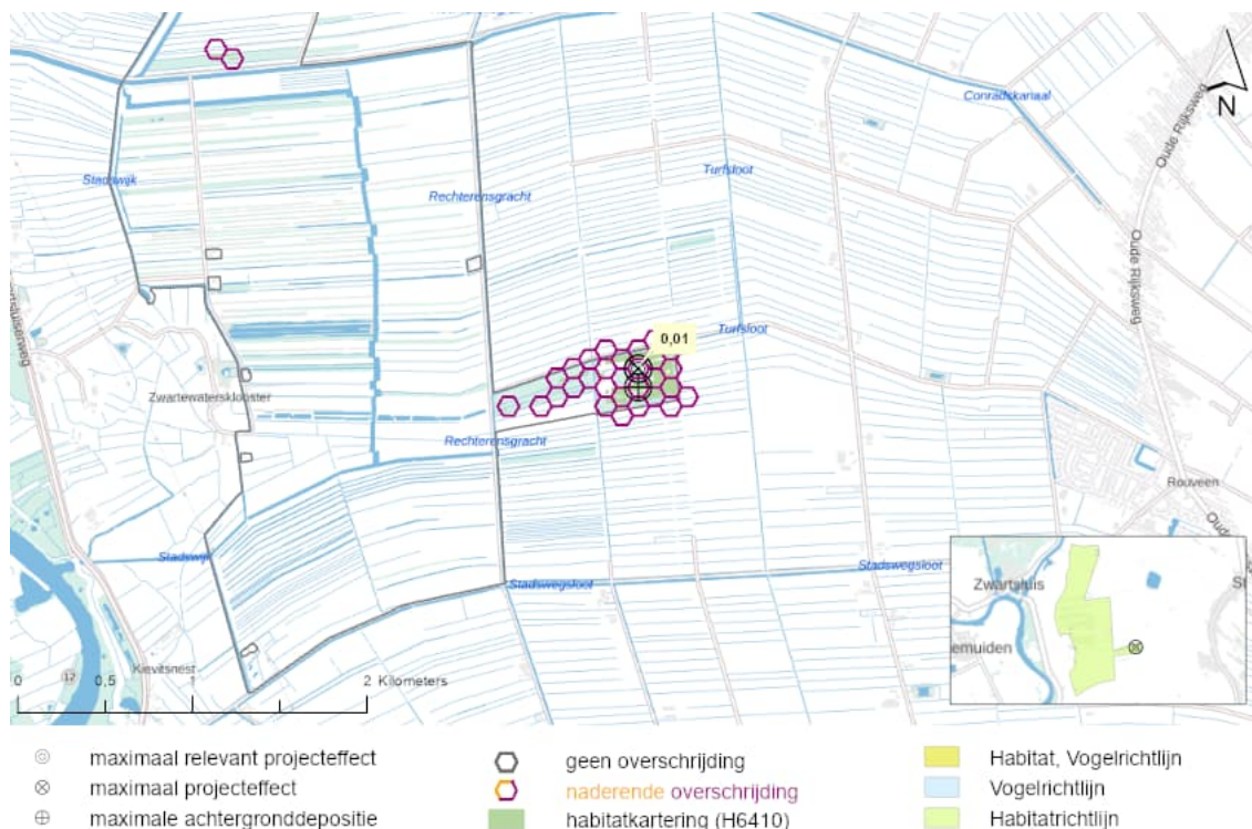
Figuur 20.3: De locatie in het Natura 2000-gebied Olde Maten & Veerslootslanden met de maximale relevante toename van stikstofdepositie op Blauwgraslanden (H6410).
