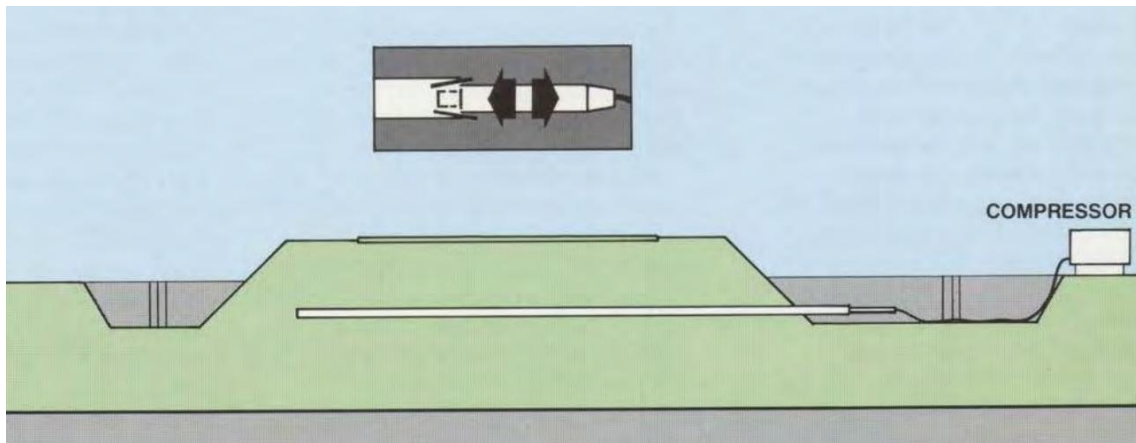
Afbeelding 5 Principeschets van de pneumatische boortechneik
