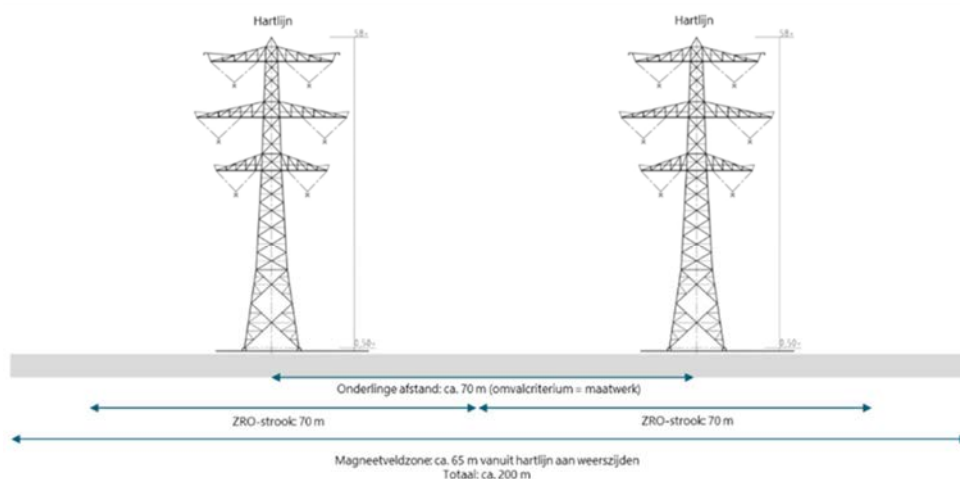
Figuur 3 Afmetingen voor dubbele mastenrij (ZRO-strook & magneetveldzone)
