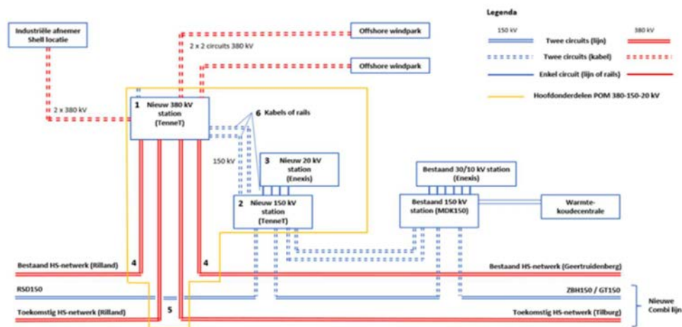
Figuur 1 Schematische weergave van de hoofdonderdelen van het voorgenomen project
