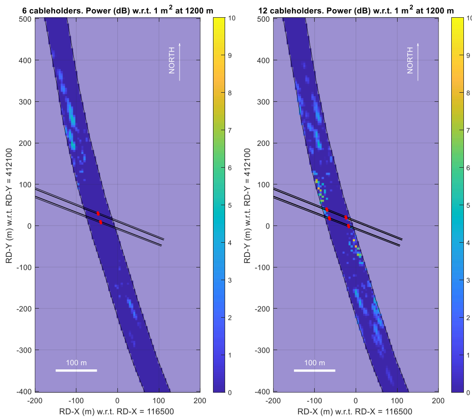
Figuur 8. Totale maximale reflectie van de combinatie van de 6 gecentreerde (links) en 12 uit het midden geplaatste (rechts) afstandhouders t.o.v. een referentiedoel met een RCS van 1 m² op 1200 m afstand. De kleurenschaal is in dB-waarden tussen 0 en 10.
