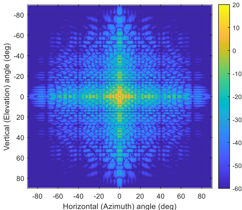
Figuur 5. RCS (dBm 2 ) van de afstandhouder als functie van aanzichtshoek. De kleurenschaal geeft de sterkte van de RCS aan van -60 dBm 2 tot 20 dBm 2 . Maximale RCS is 18 dBm 2 oftewel 67 m 2 .
