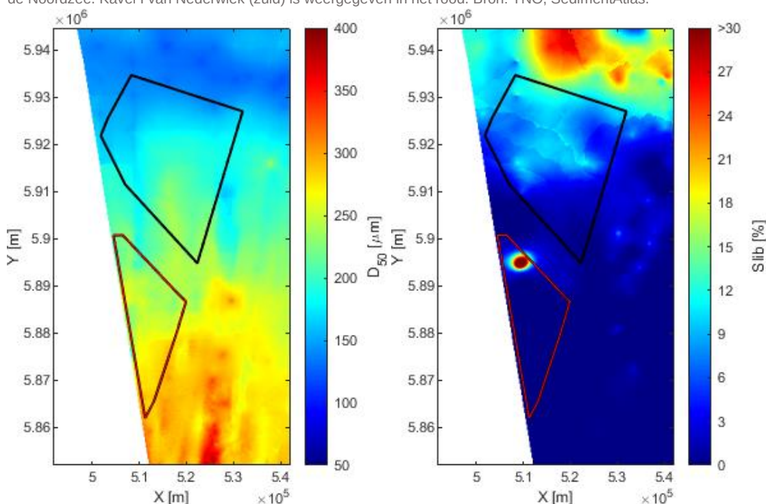
Figuur 5.8 Mediane korreldiameter ( D_{50} ) links en percentage slib van het sediment in de bovenste laag van de bodem op de Noordzee. Kavel I van Nederwiek (zuid) is weergegeven in het rood. Bron: TNO, SedimentAtlas.
