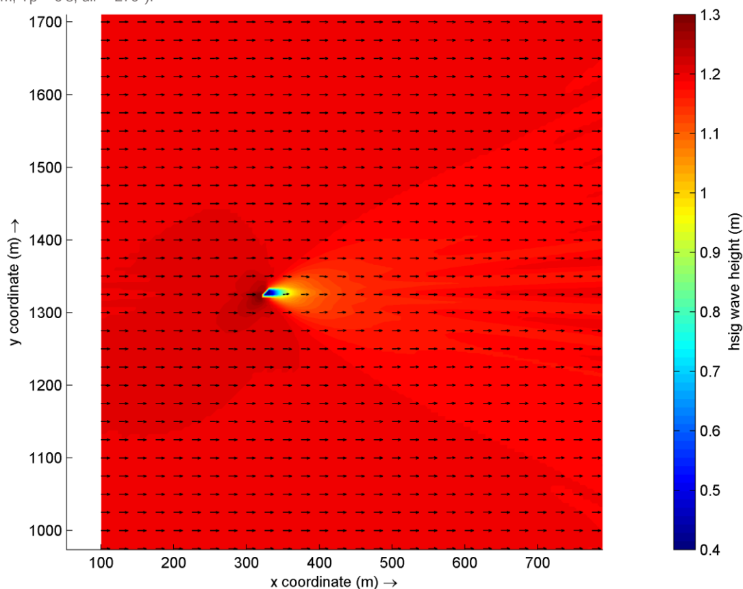
Figuur 5.13 SWAN modelresultaat: effect van een paal met een diameter van 10 m op het inkomende golfveld ( H_s = 1,2 m, T_p = 6 s, \text{dir} = 270^\circ ).
