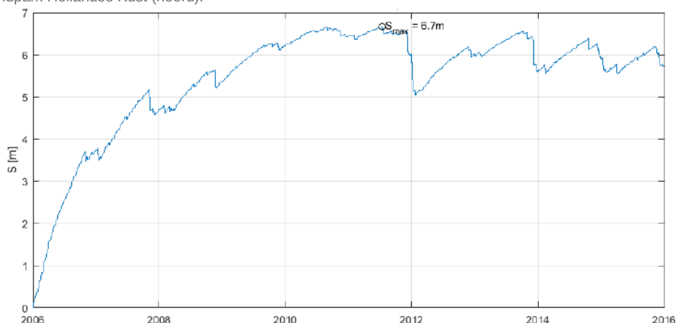
Figuur 5.20 Gemodelleerde ontwikkeling van de diepte van een ontgrondingskuil (S) in de tijd voor een fundering in het windpark Hollandse Kust (noord).
