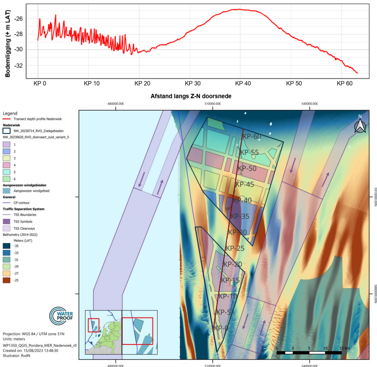
Figuur 5.7 Bovenste paneel: doorsnede van de bodemligging in het windenergiegebied Nederwiek van zuid naar noord. Onderste paneel: locatie van de doorsnede inclusief kilometrerings (KP = kilometerpunt).
