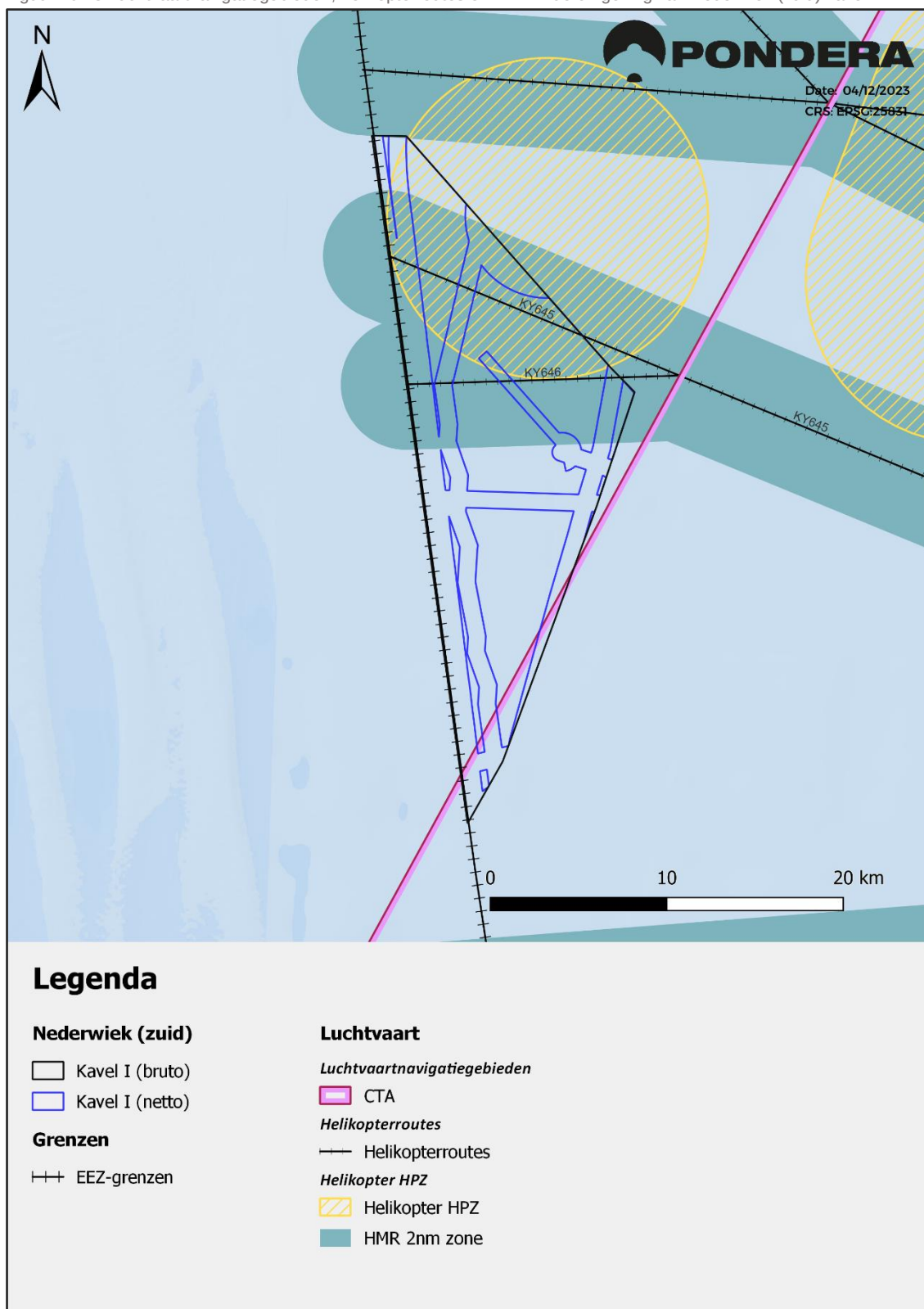
Figuur 10.13 Luchtvaarnavigatiegebieden, helikopterroutes en HPZ in de omgeving van Nederwiek (zuid) kavel I
