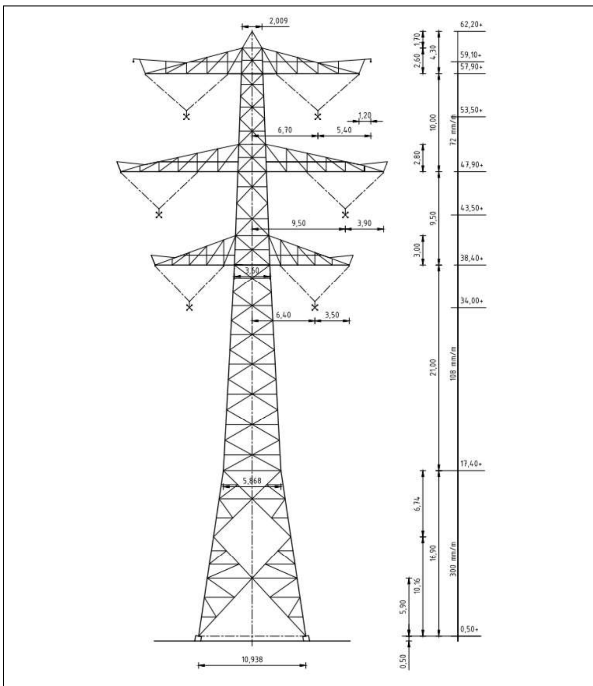
Figuur 4 Mastbeeld masttype S+6/s
