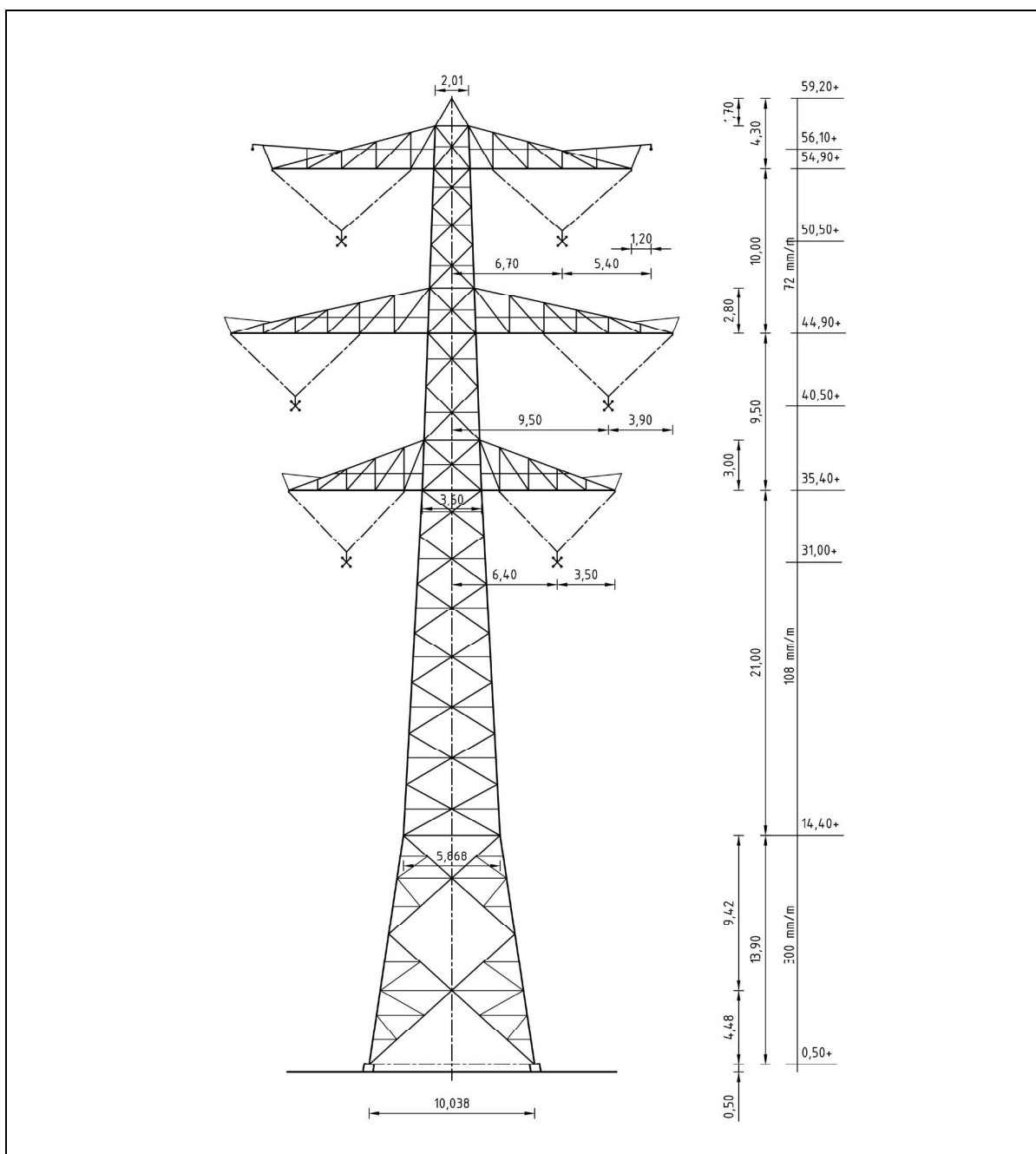
Figuur 3 Mastbeeld masttype S+3/s
