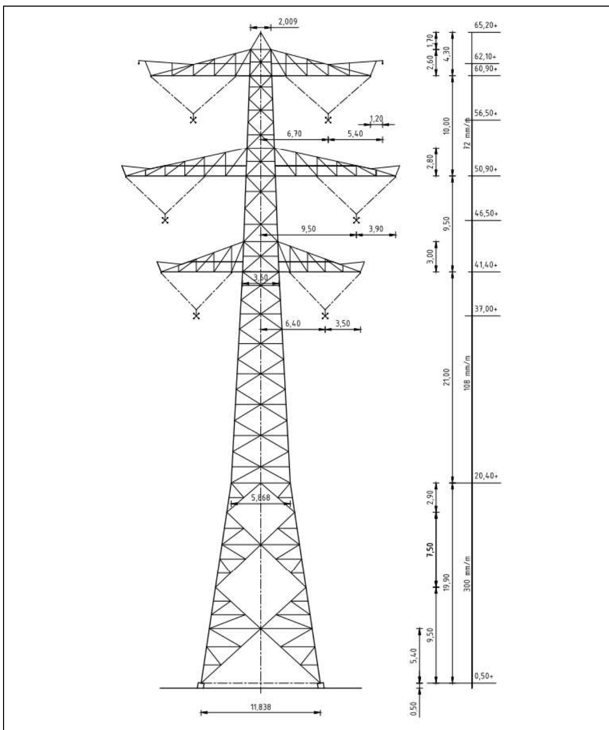
Figuur 5 Mastbeeld masttype S+9/s
