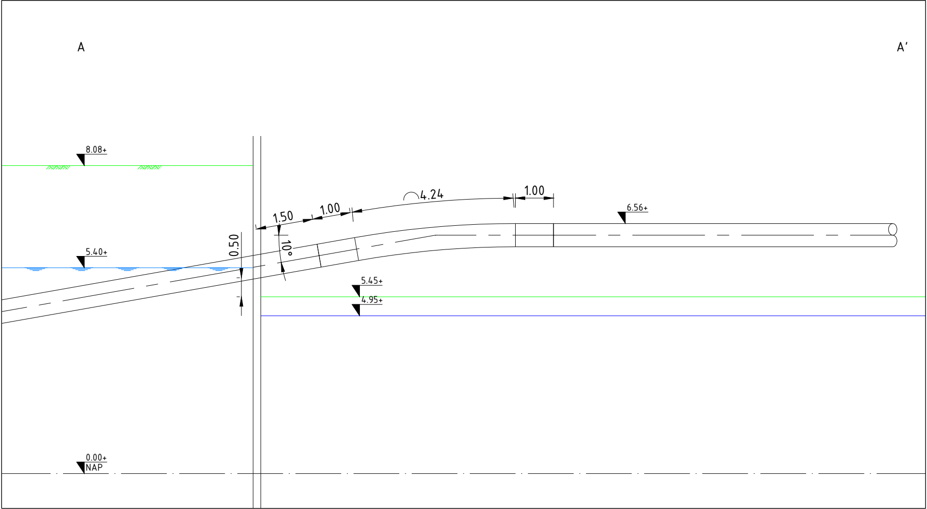
Aanzicht-DWP-01, schaal : 1-100
