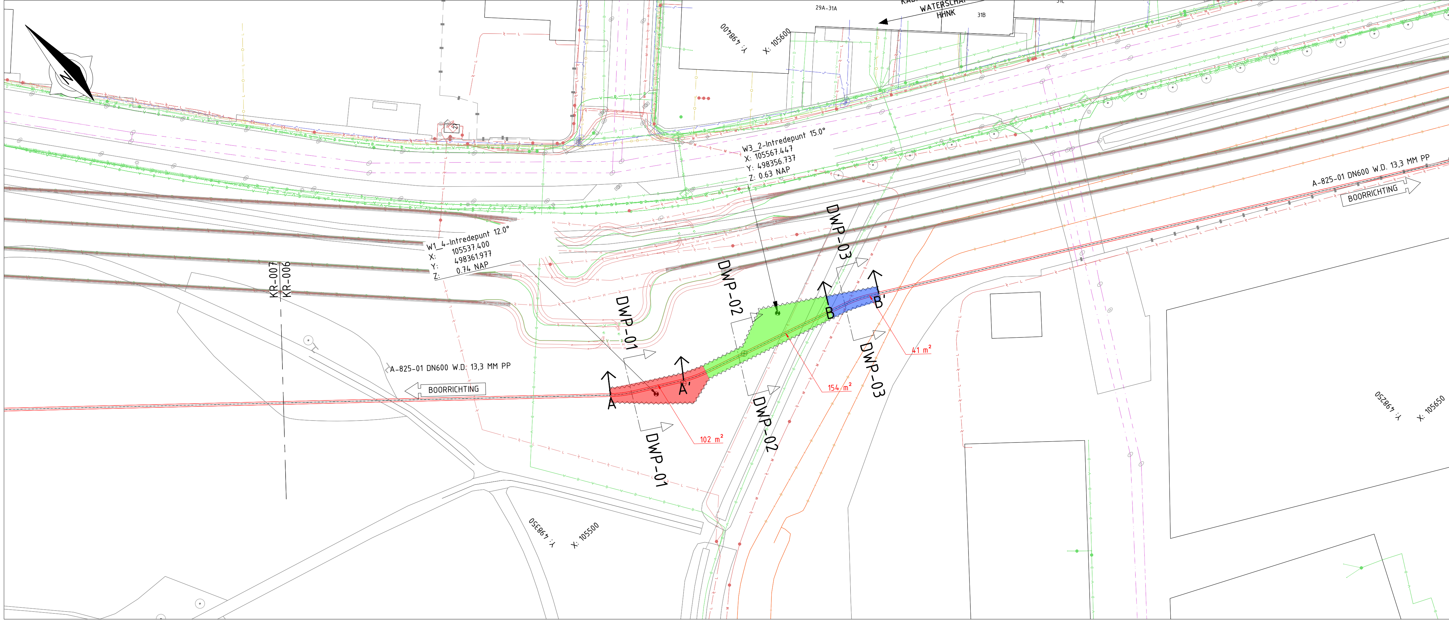
Bovenaanzicht, Schaal : 1-500
