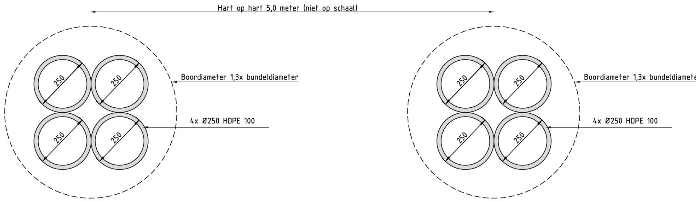
Doorsnede bundel HDD SCHAAL 1 : 10 in mm
