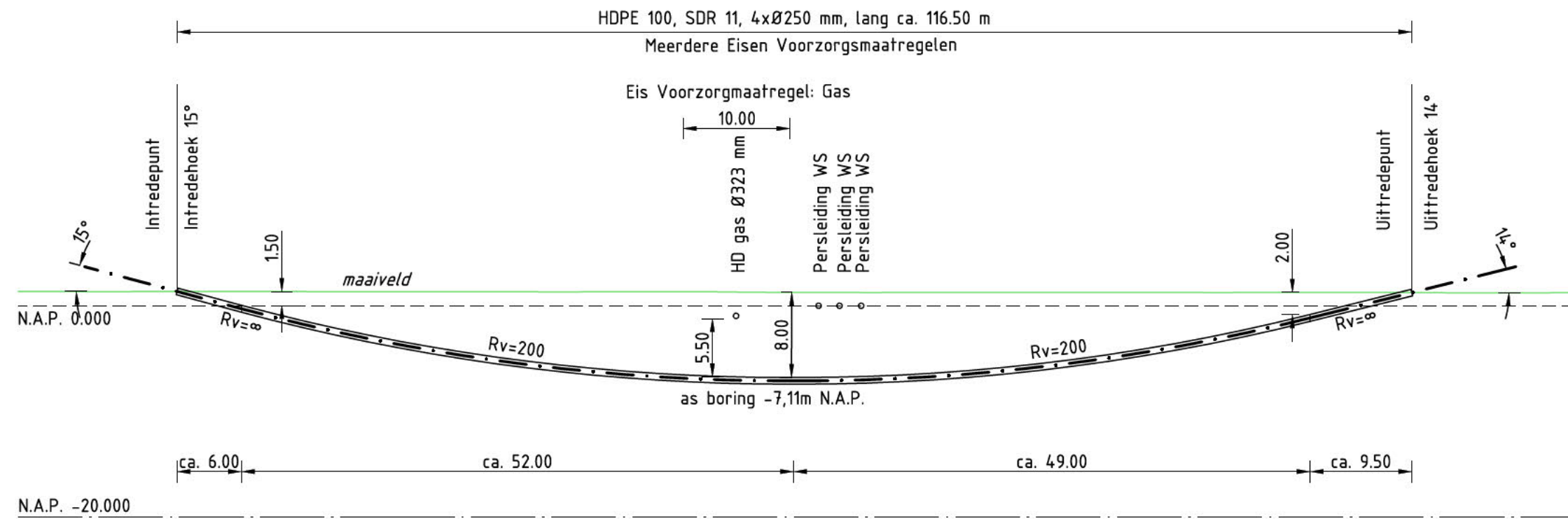
Lengte profiel boring HDD onder leidingen (N16) DWP A-A' SCHAAL 1 : 500 (Lengte profiel gegenereerd uit de AHN3)
