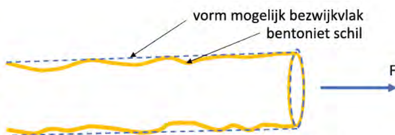
Figuur 4.2 Schematische weergave langsrichting bezwijkvlak langs bentoniet.
