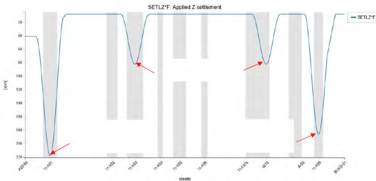
Figuur 2.8: Weergave uitvoeringszakkingen RK11 in het rekenmodel (inclusief zettingen, onzekerheids- en belastingfactor)
