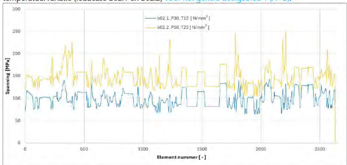
Figuur 3.11: Von Mises spanning op basis van druk- en temperatuurvariatie voor deelgebied 1 (Blauwe lijn: Druk = 30 bar & T = 15°C; Oranje lijn: Druk = 50 bar & T = 25°C).
