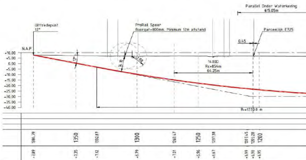
Figuur 3.8: NEN3651 veiligheidszone voor de westelijke zijde van HDD BUKO. Uittredpunt op ruim 150 m
