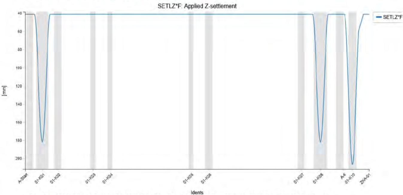
Figuur 2.6: Weergave uitvoeringszakkingen RK1 in het rekenmodel (inclusief zettingen, onzekerheids- en belastingfactor)
