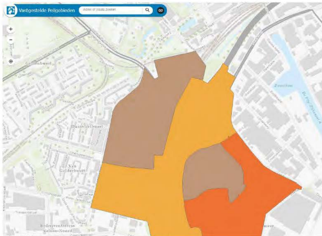
Figuur B5-1: Peilgebied watrgang ten westen van intredepunt
