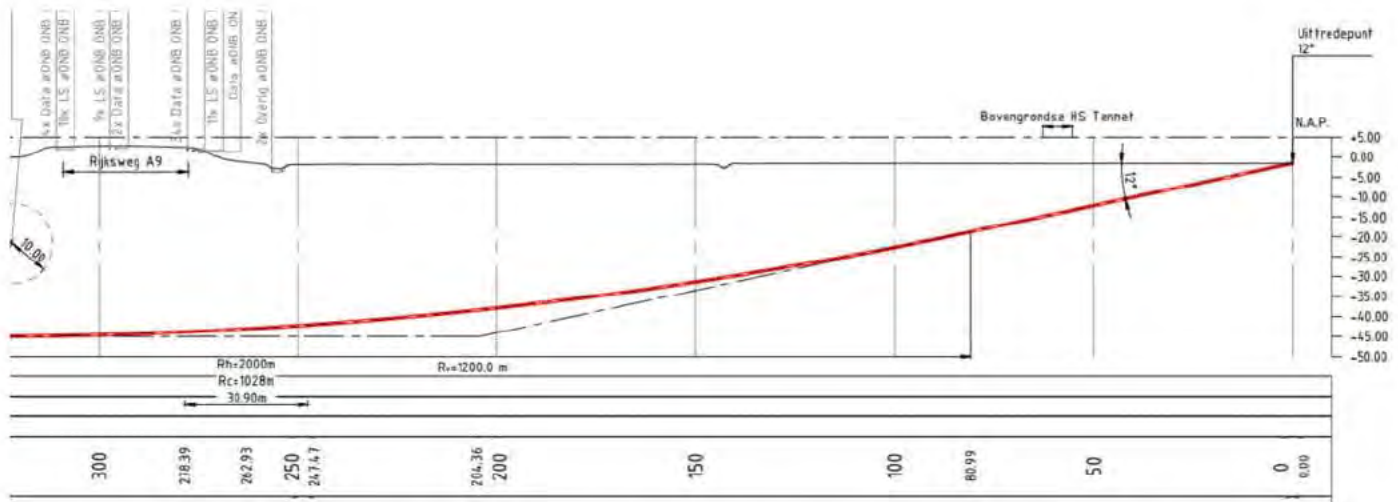
Figuur 3.3: NEN3651 veiligheidszone voor de oostelijke zijde van HDD Zijkanaal A. Uittredepunt op ruim 200 m
