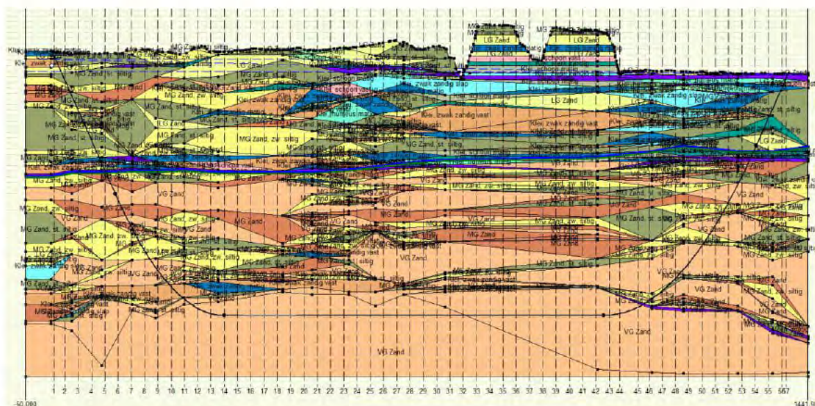
Aan de hand van de grondonderzoeken is een bodemprofiel opgesteld over de boortlijn. In het volgende figuur is de vastgestelde grondopbouw zichtbaar.
