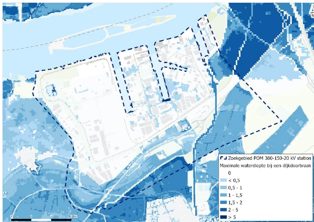
Afbeelding 6.1 Overstromingsrisico zoekgebied POM 380-150-20 kV in meters
