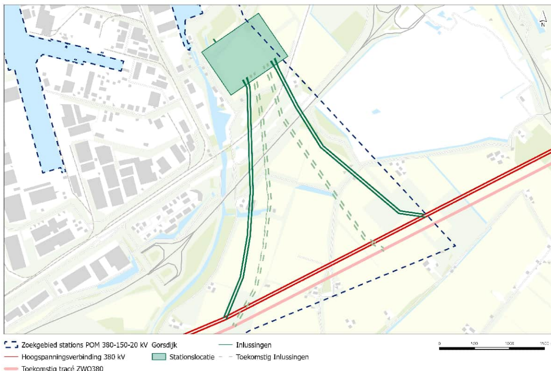
Afbeelding 2.7 Overzicht van het onderzoeksalternatief Gorsdijk; met de 380 kV-verbindingen en indicatieve inlissingen op het toekomstige en bestaande hoogspanningsnetwerk ingetekend
