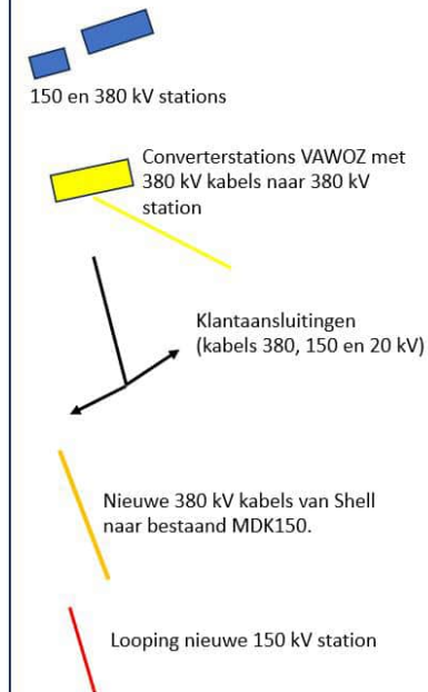
Zoekgebied Keeneweg (Locatie-optie 4)
