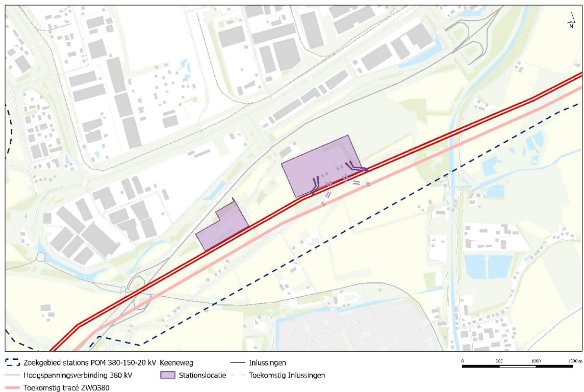
Afbeelding 2.5 Overzicht van het onderzoeksalternatief Keeneweg; met de 380 kV-verbindingen en indicatieve inlusingen op het toekomstige en bestaande hoogspanningsnetwerk ingetekend
