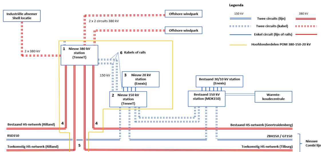
Afbeelding 1.1 Schematische weergave van de hoofdonderdelen van POM 380-150-20 kV, weergegeven binnen de bredere invalshoek van de IEA. De getallen bij de onderdelen refereren naar de opsommingennummers in de bovenstaande tekst
