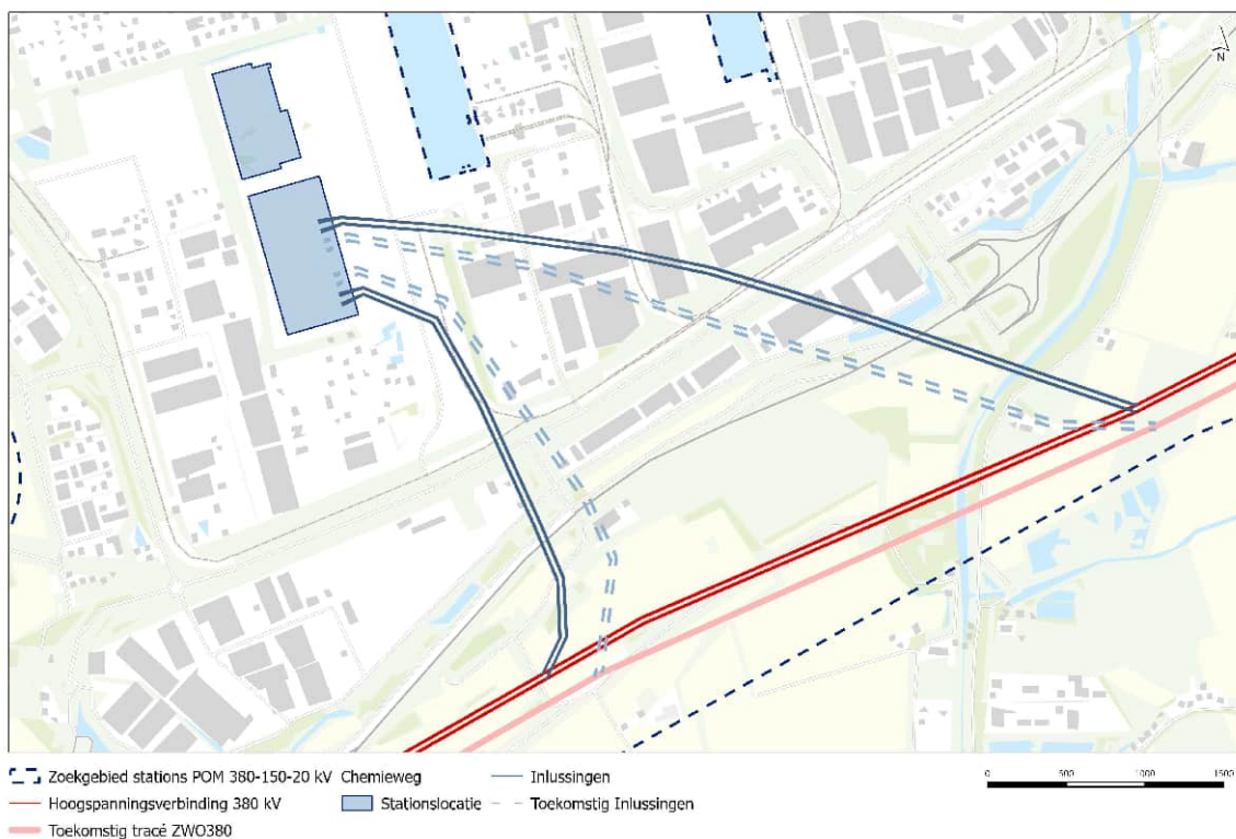
Afbeelding 2.3 Overzicht van het onderzoeksalternatief Chemieweg; met de 380 kV-verbindingen en indicatieve inlussen op het toekomstige- en bestaande hoogspanningsnetwerk ingetekend
