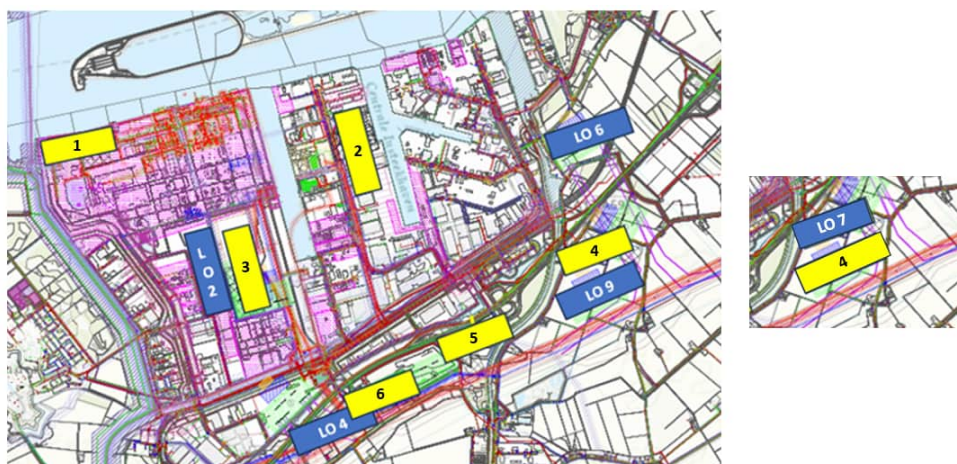
Afbeelding 6.2 Kaartweergave met VAWOZ converterlocatie-opties (gele blokjes) en de stationslocaties voor de hoogspanningsstations (blauwe blokjes)
