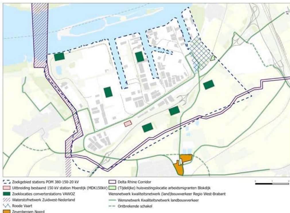
Afbeelding 8.1 Raakvlakprojecten in en rond het zoekgebied voor POM 380-150-20 kV
