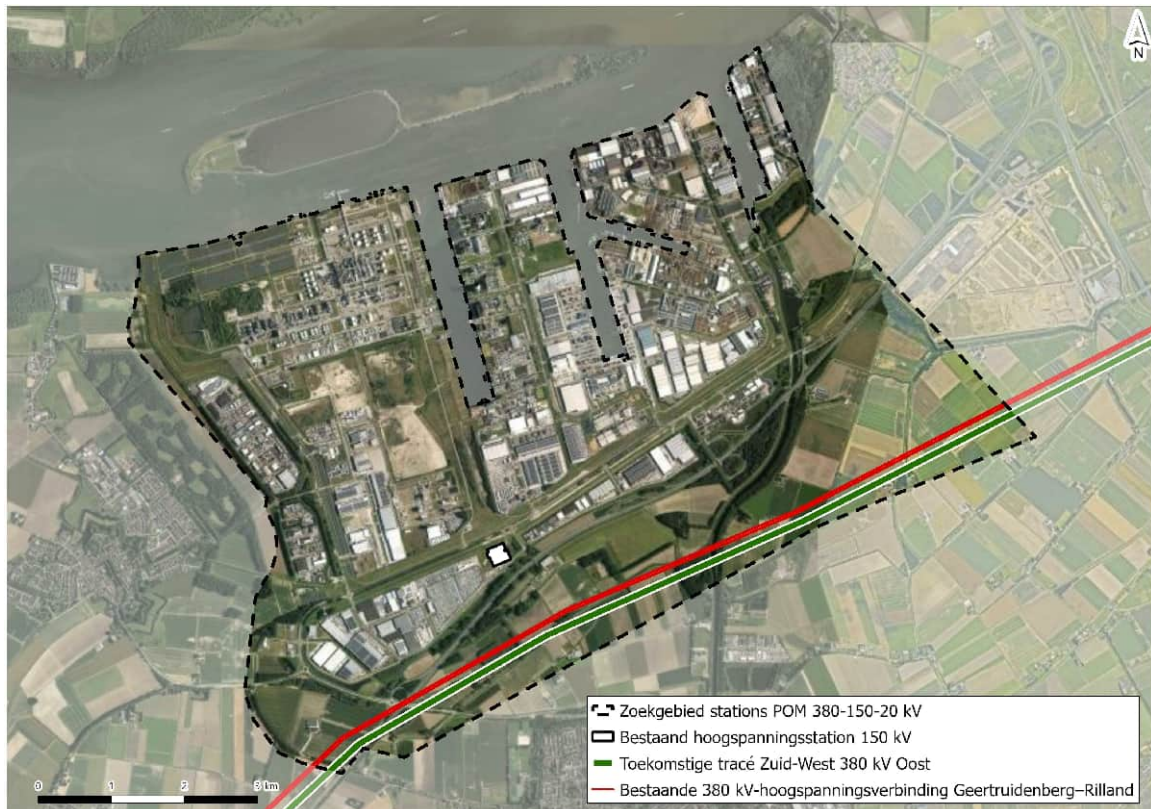
Afbeelding 1.2 Luchtbeeld van het zoekgebied voor POM 380-150-20 kV
