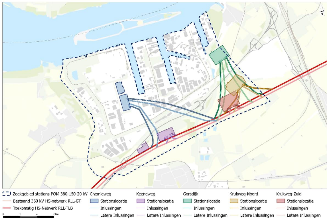
Afbeelding 2.2 Overzicht met de onderzoeksalternatieven (stationslocaties en inlussingen) voor POM 380-150-20 kV
