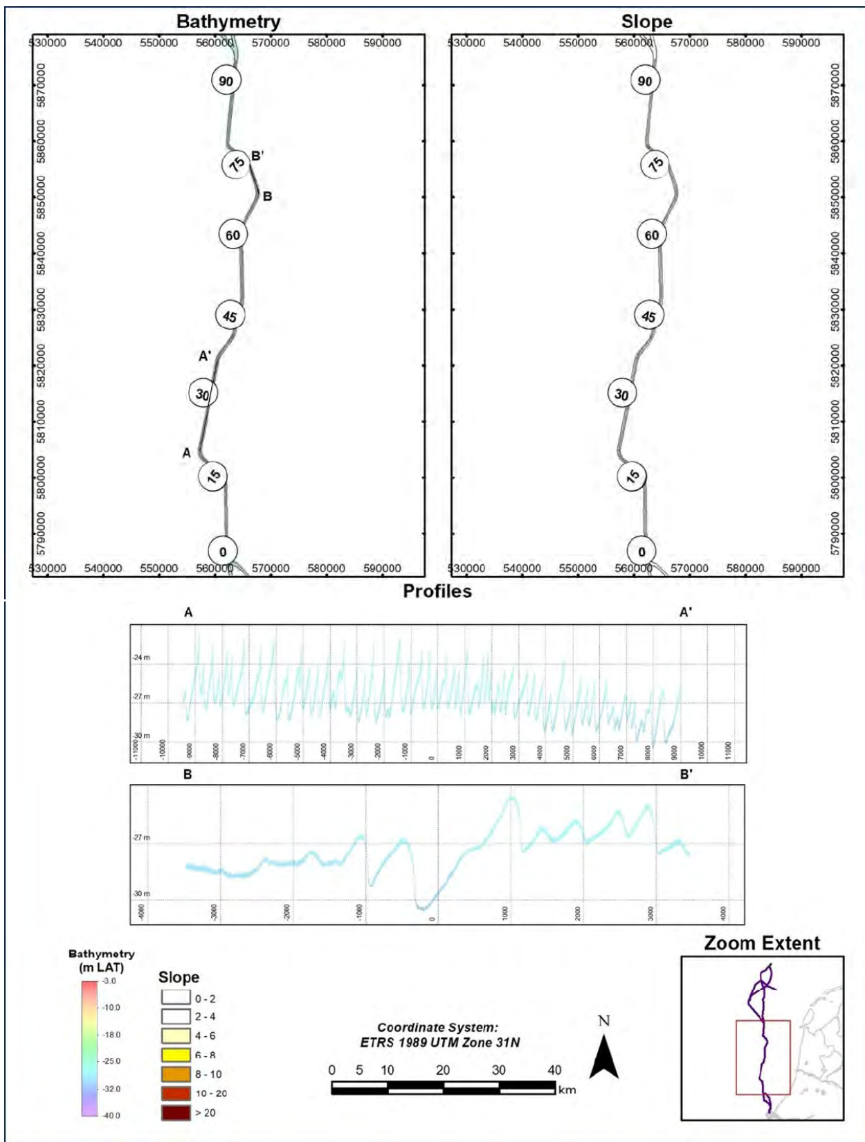
Figuur 4-8 – Zeebodem sectie A-A' met zandgolven (Fugro rapport)
