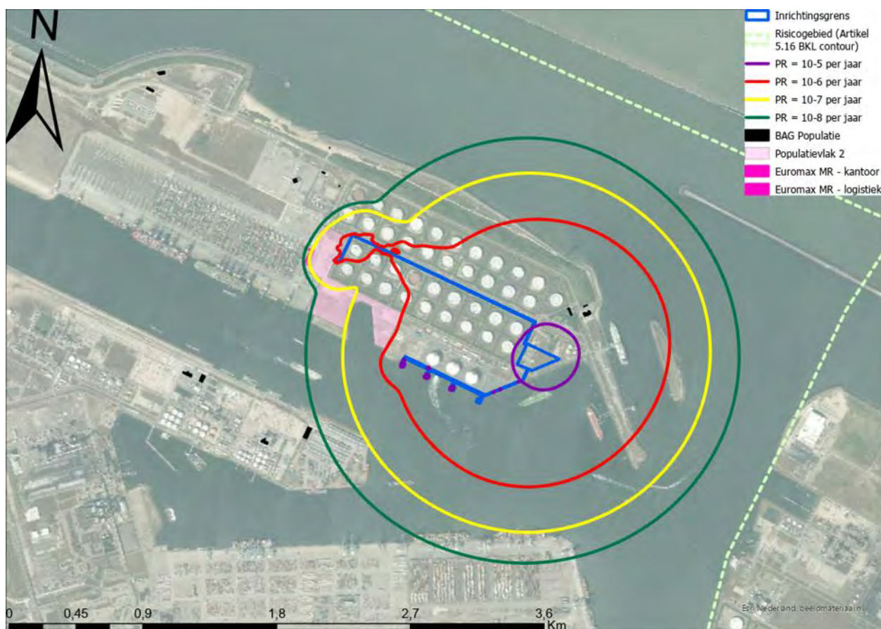
Figuur 8-4 PR-contouren voor het MOT terminalalternatief met spheres..
