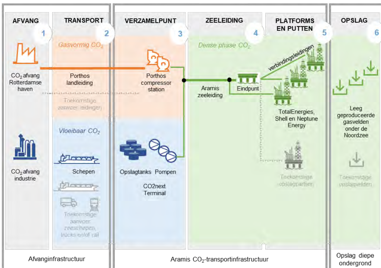
Figuur 1-3. Schematisatie van de onderdelen van de integrale CCS-keten. Aramis levert daarvoor de CO 2 transportinfrastructuur inclusief drie platforms met verbindingssleidingen.
