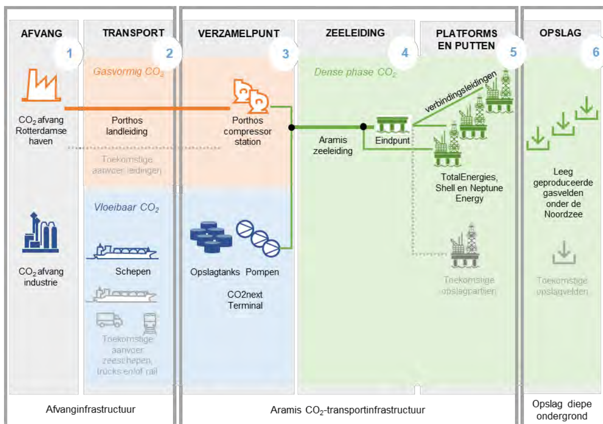
Figuur 3-1: Schematisatie van de onderdelen van de integrale CCS-keten. Aramis levert daarvoor de CO 2 transportinfrastructuur inclusief drie platforms met verbindingssleidingen.
