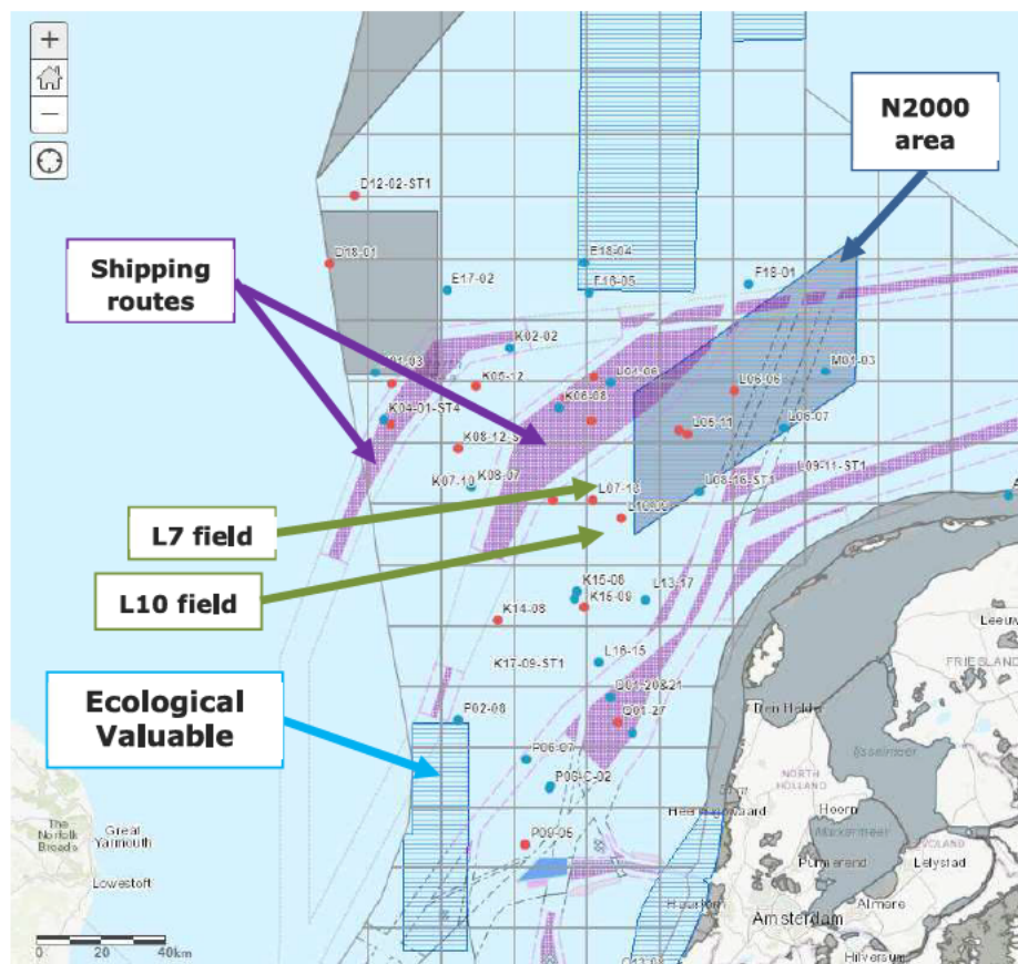
Figuur: Ligging van het L7 en het L10 veld t.o.v. bijzondere gebieden
