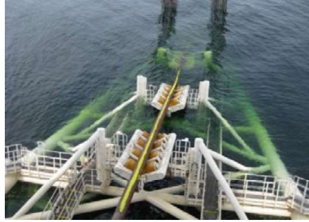
Figuur: Verwijderen van pijpleidingen met behulp van reverse S-Lay
