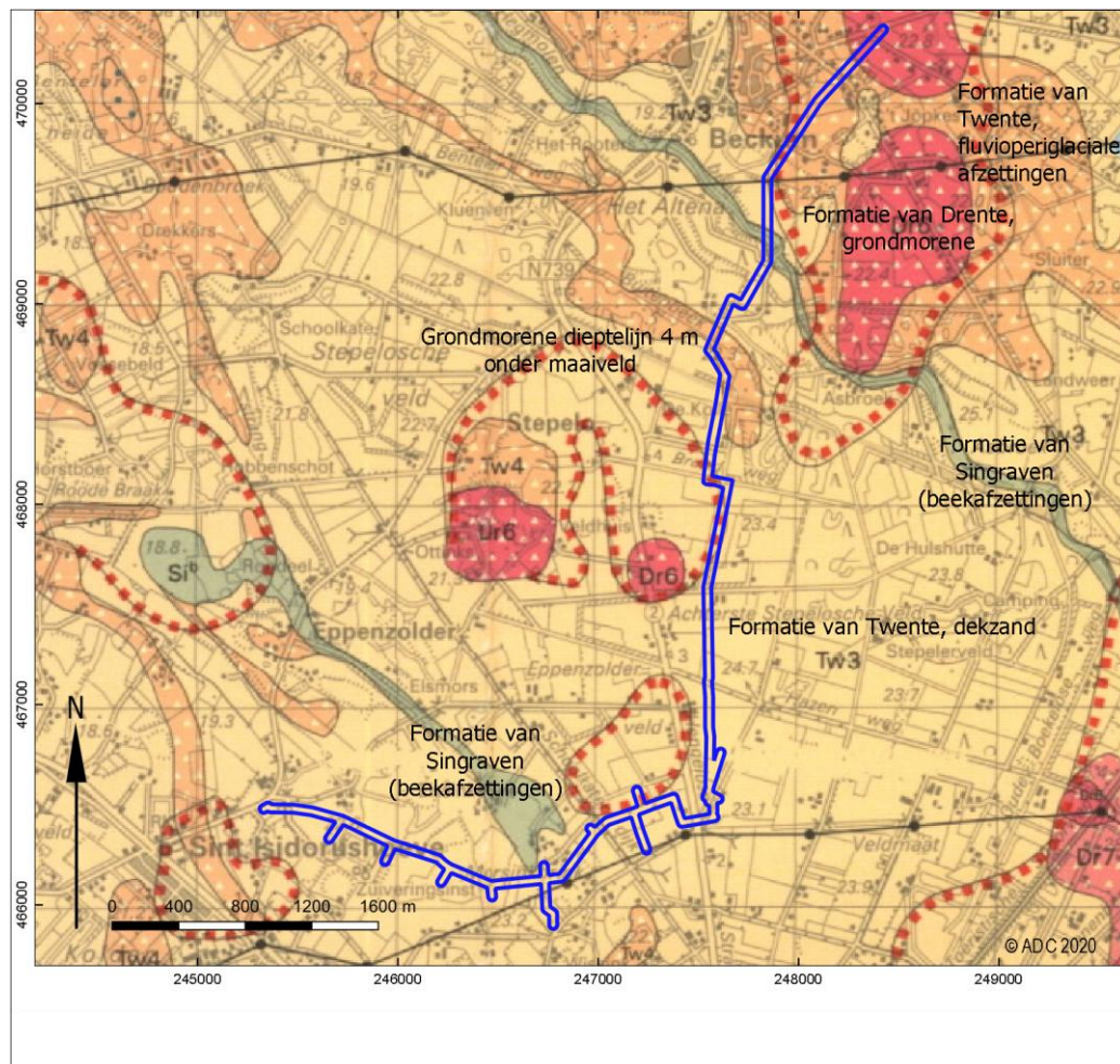
Afb. 7 Geologische kaart
