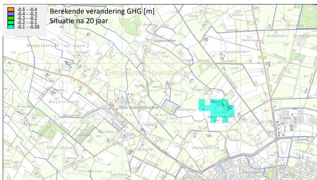
Figuur 4.1: Berekende effect op de GHG
