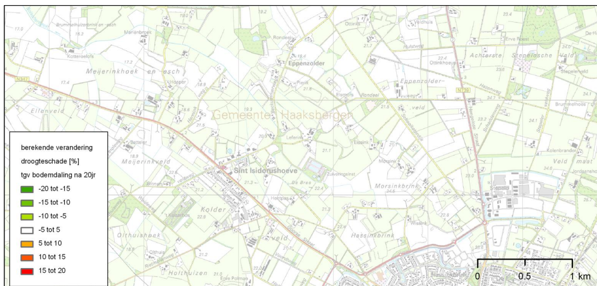
Figuur 4.5: Berekende verandering droogteschade
