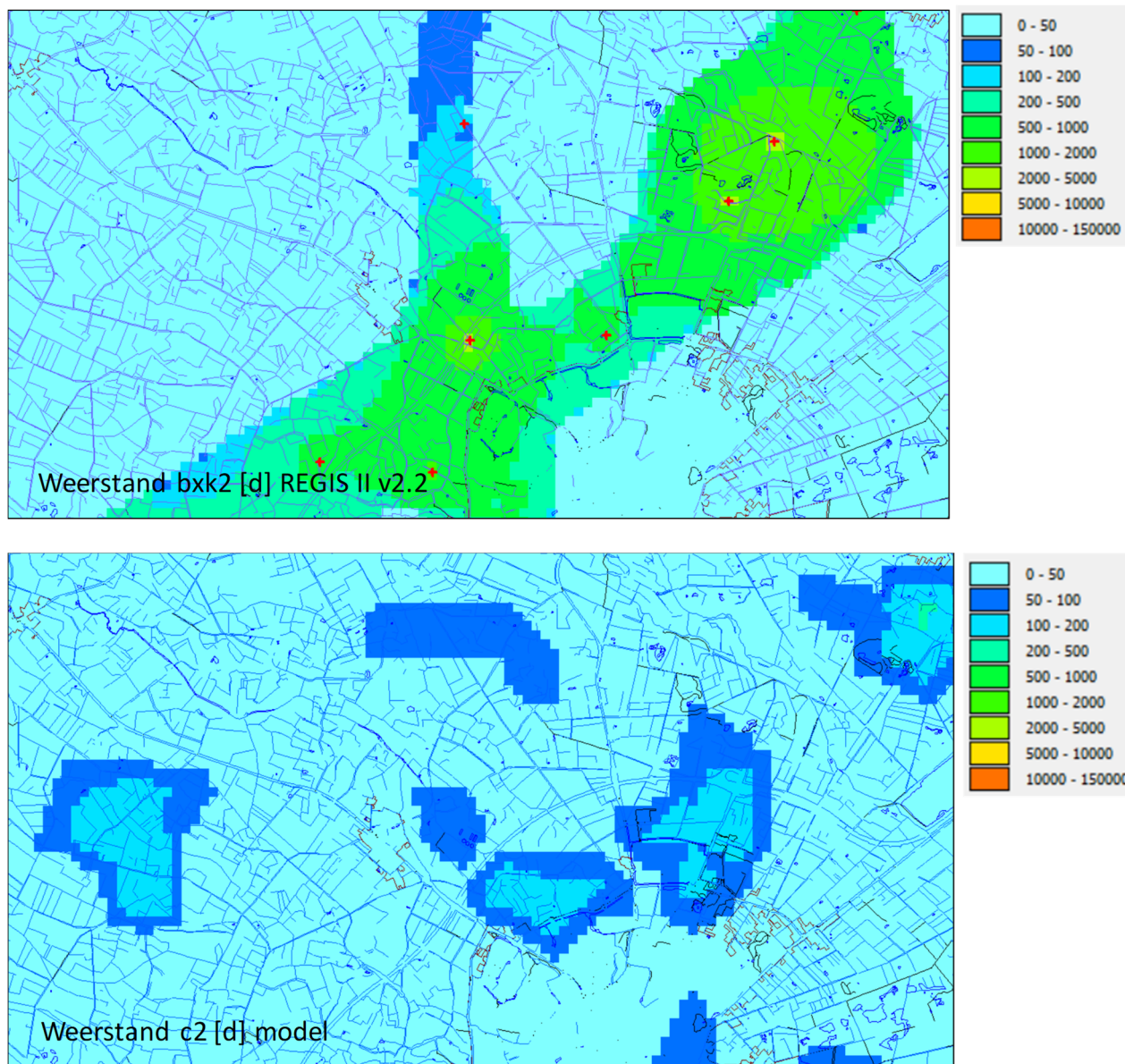
Figuur B2..2 Weerstand bxx2 in REGIS II v2.2 (boven) en weerstand in het model (onder). Locaties van boringen waar de schematisatie op gebaseerd is, zijn weergegeven met een rood plusteken.
