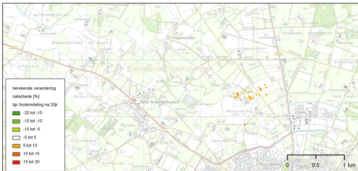
Figuur 4.4: Berekende verandering natschade
