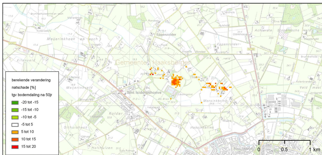
Figuur 4.12: Berekende verandering natschade
