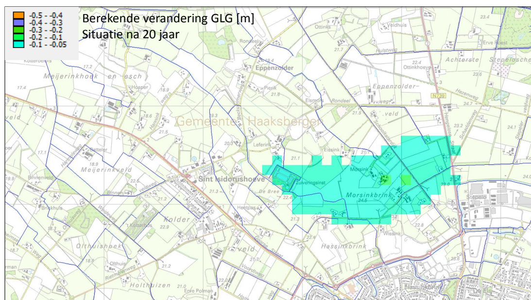
Figuur 4.2 Berekende effect op de GLG
