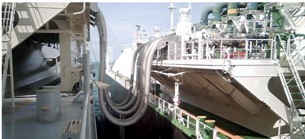
Figuur 2-3 Bovenstaande afbeelding laat zien hoe LNG van de LNG-carrier (rechts op de afbeelding) naar de FSRU (links op de foto) wordt getransporteerd met flexibele slangen
