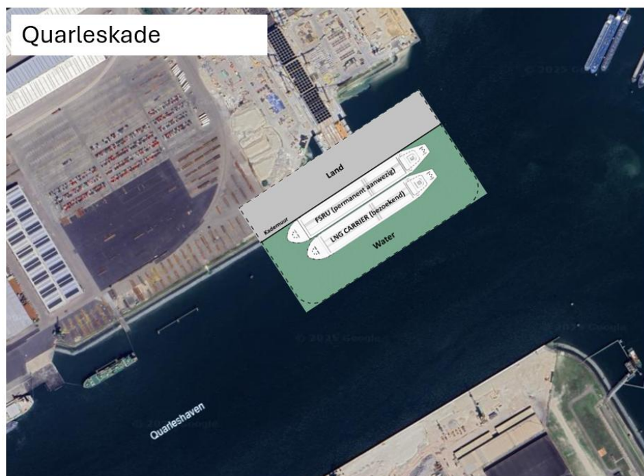
Figuur 9-2 Indicatieve layout locatie Quarleskade North
