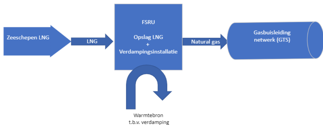
Figuur 2-3 Een globaal processchema (bron: VTTI)
