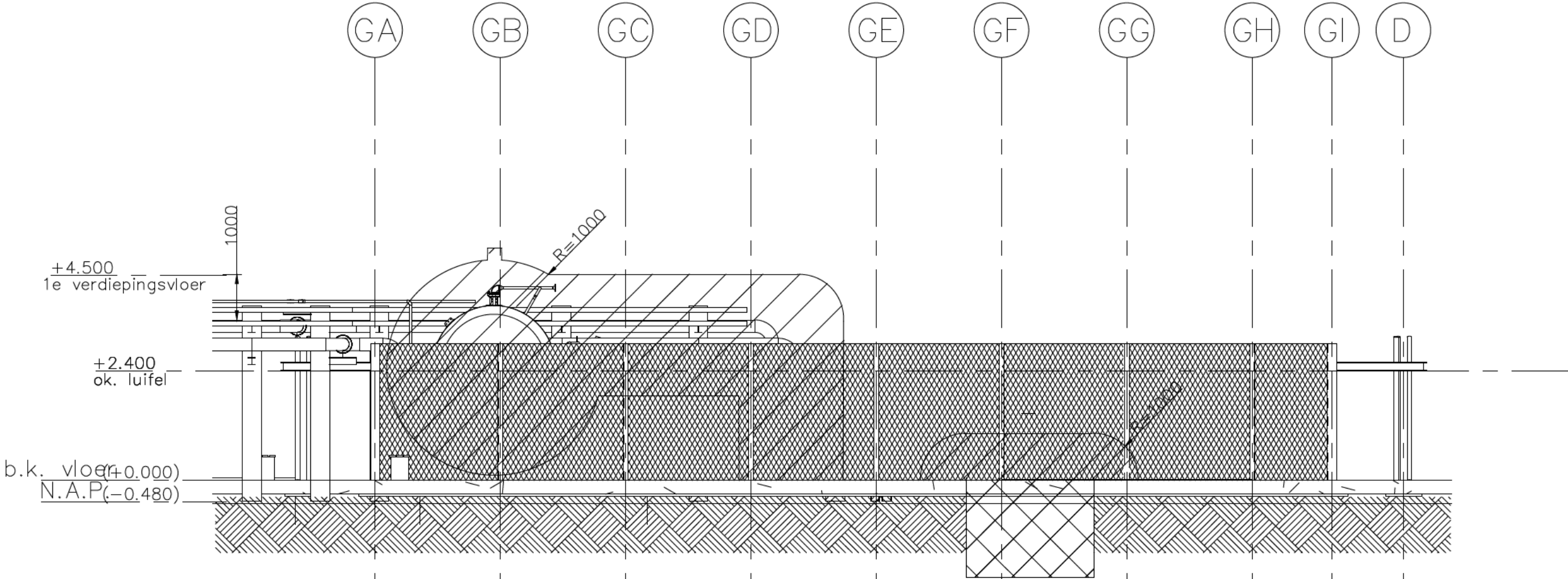
Vooraanzicht boorlocatie Schaal: 1 : 100
