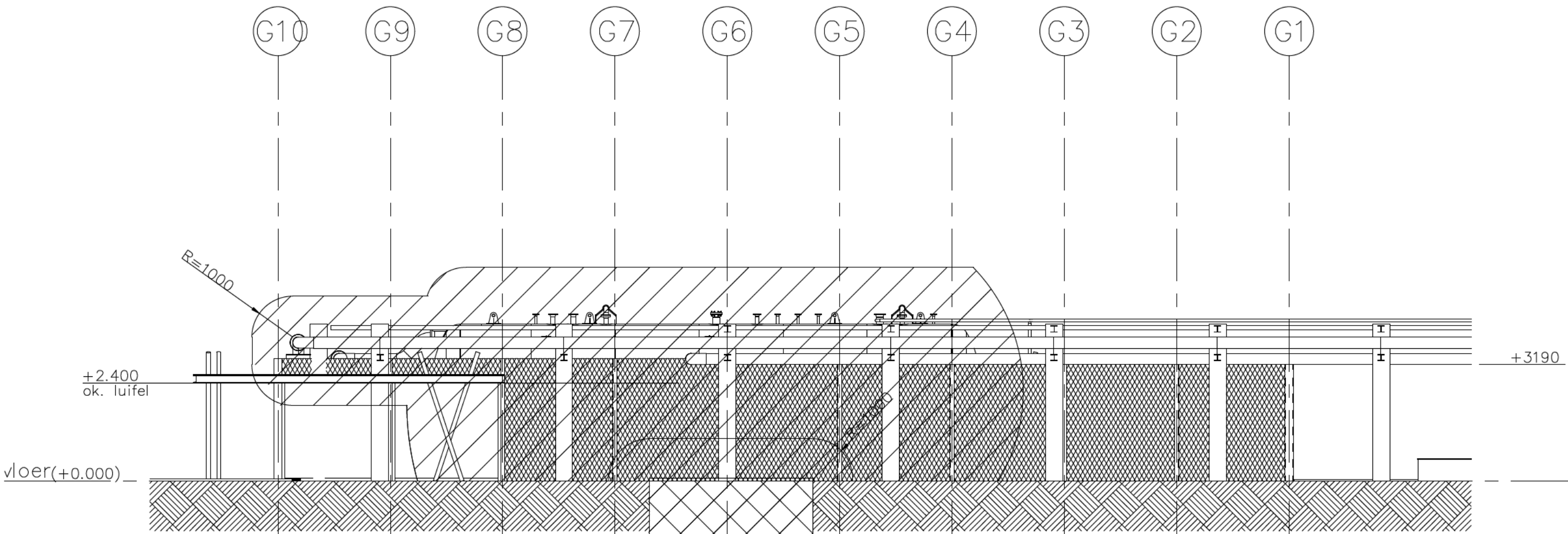
Linkezijanzicht boorlocatie Schaal: 100
