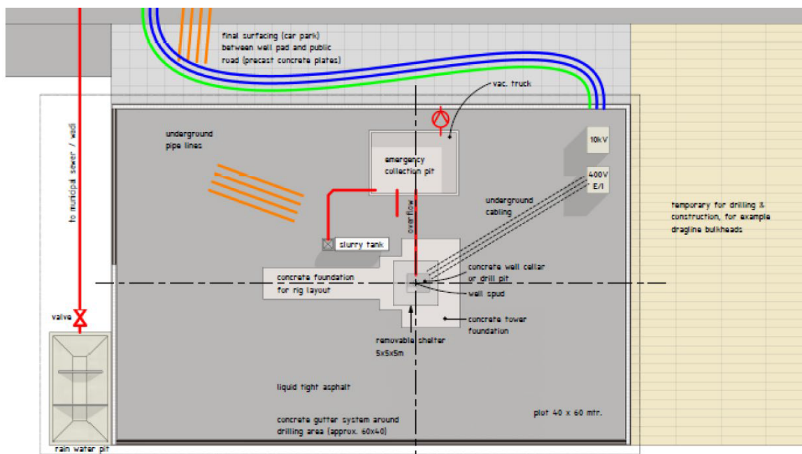
Figuur 1: Principe ontwerp van de zoutwinningslocatie
