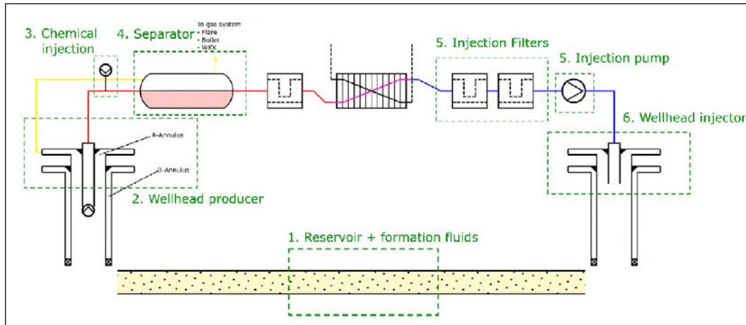
Figuur 2.3: Indicatief processchema primair circuit
