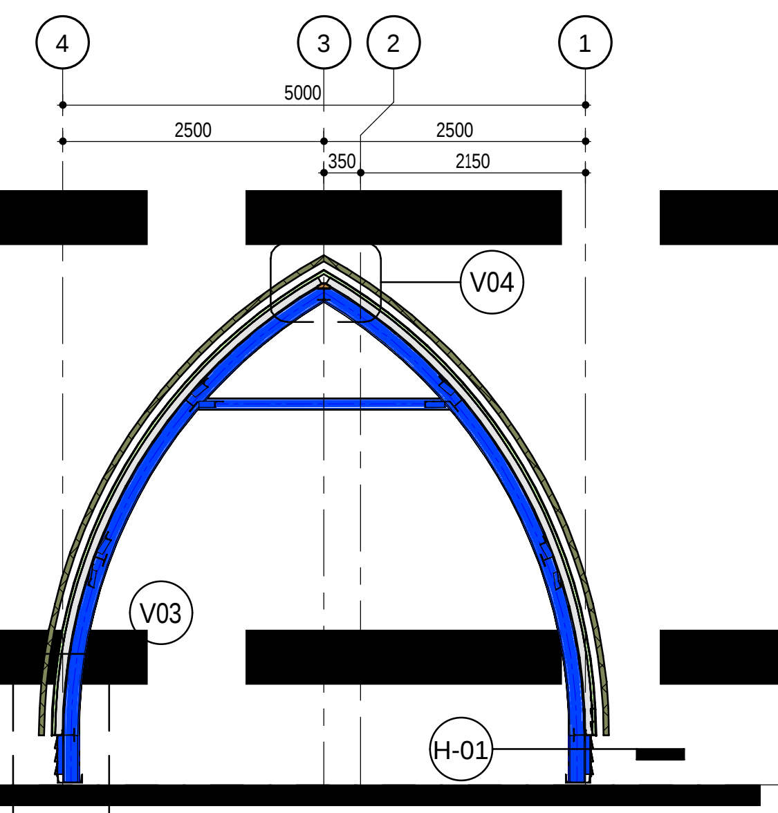
SECTION GRID B 1 : 50
