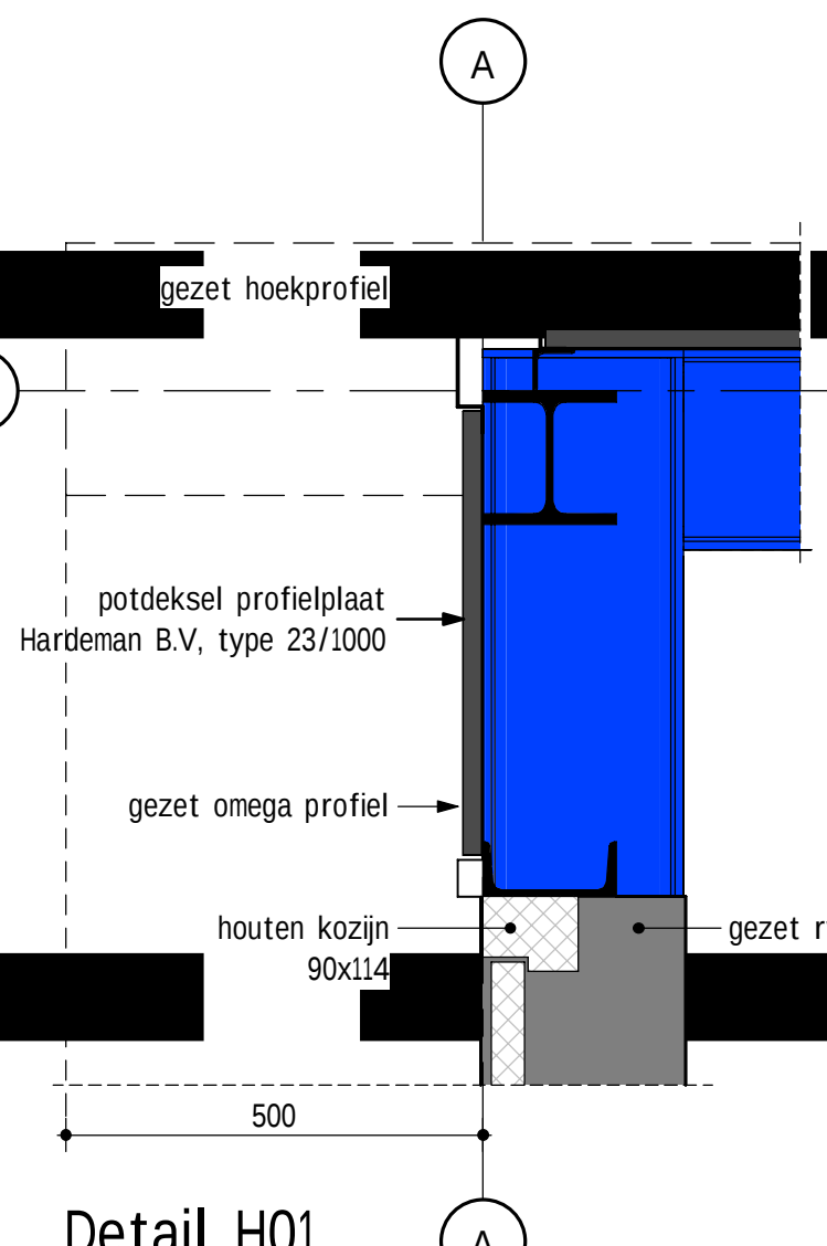
Detail H01 1 : 10
