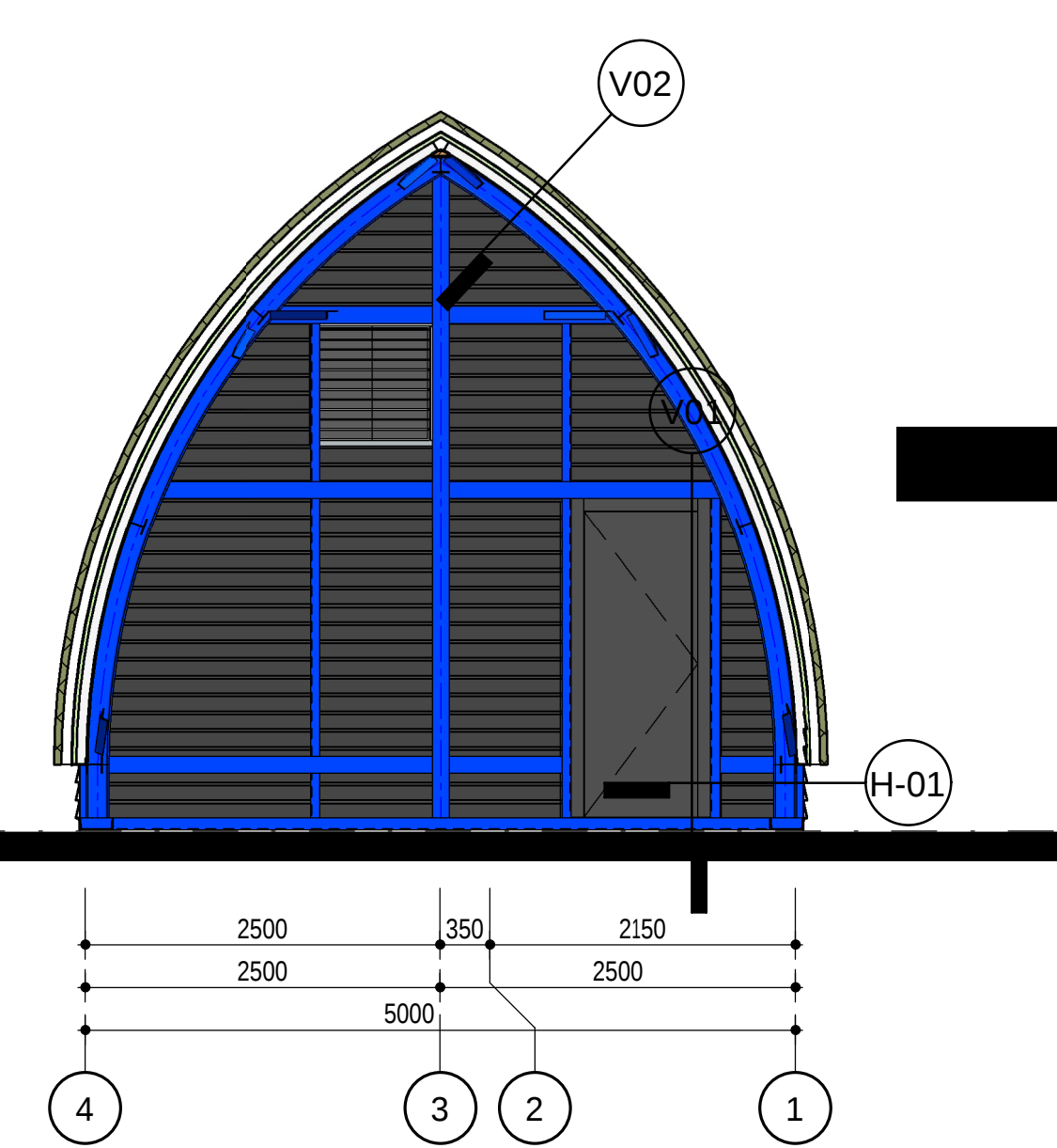
SECTION GRID 1 1 : 50
