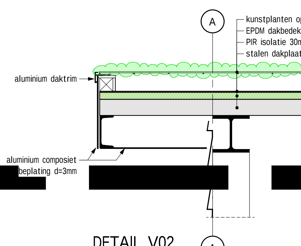
DETAIL V02 1 : 10
