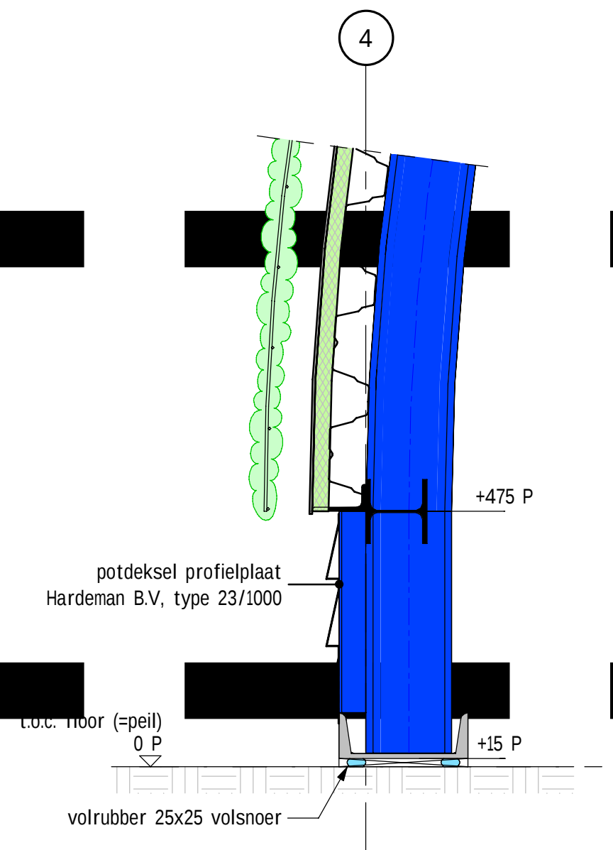
DETAIL V03 1 : 10
