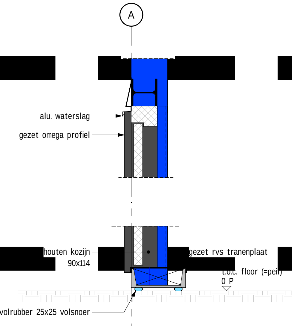
Detail V01 1 : 10
