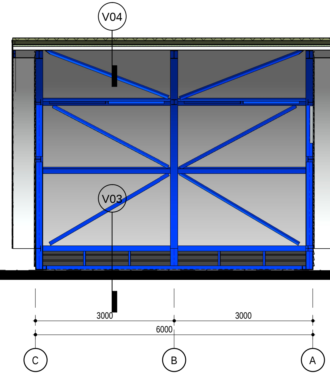
SECTION GRID 3 1 : 50
