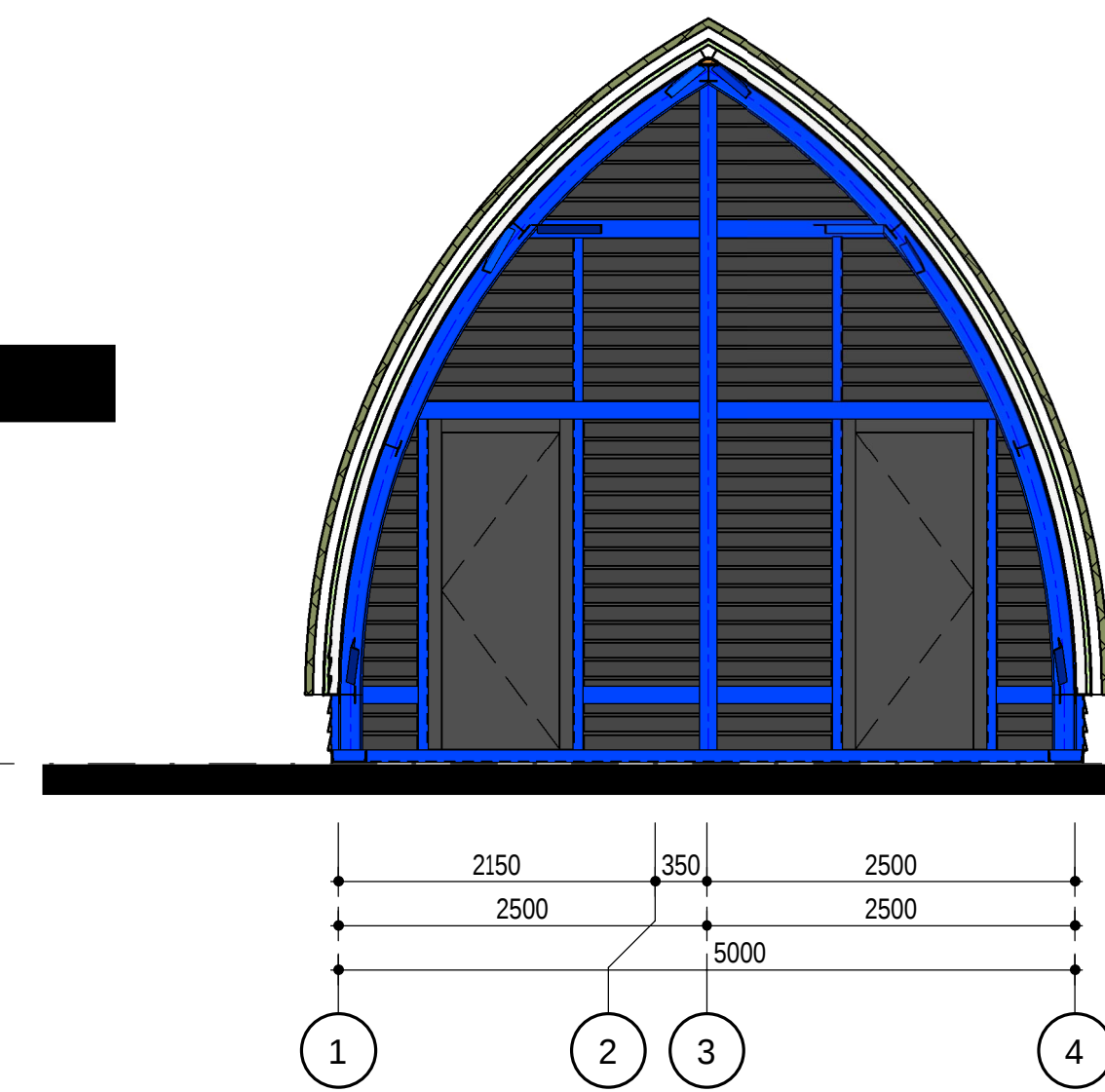
SECTION GRID C 1 : 50
