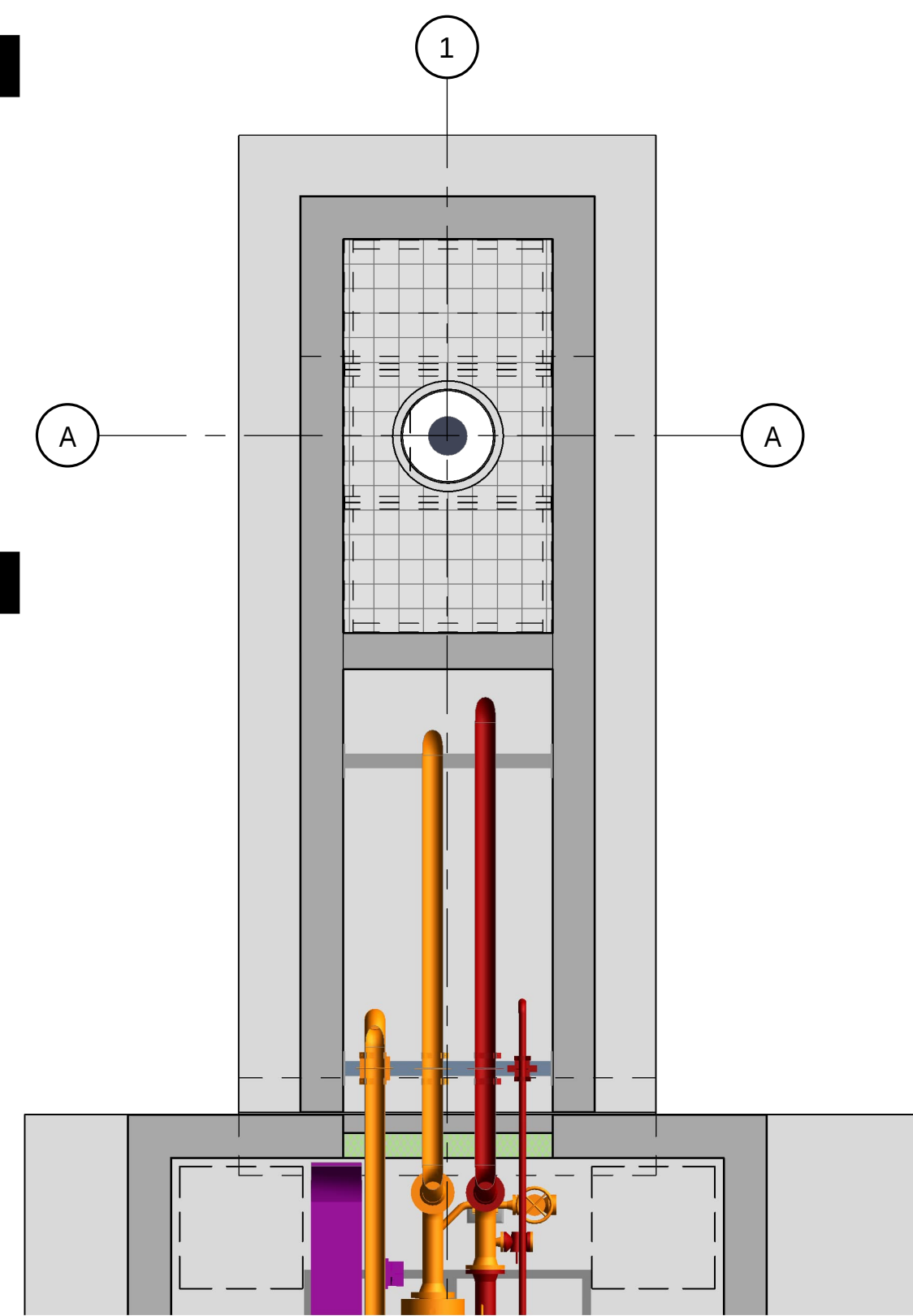
CELLAR, -1600 P 1 : 50
