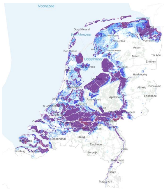
Figuur E.26: Zeer kleine kans – maximale waterdiepte
