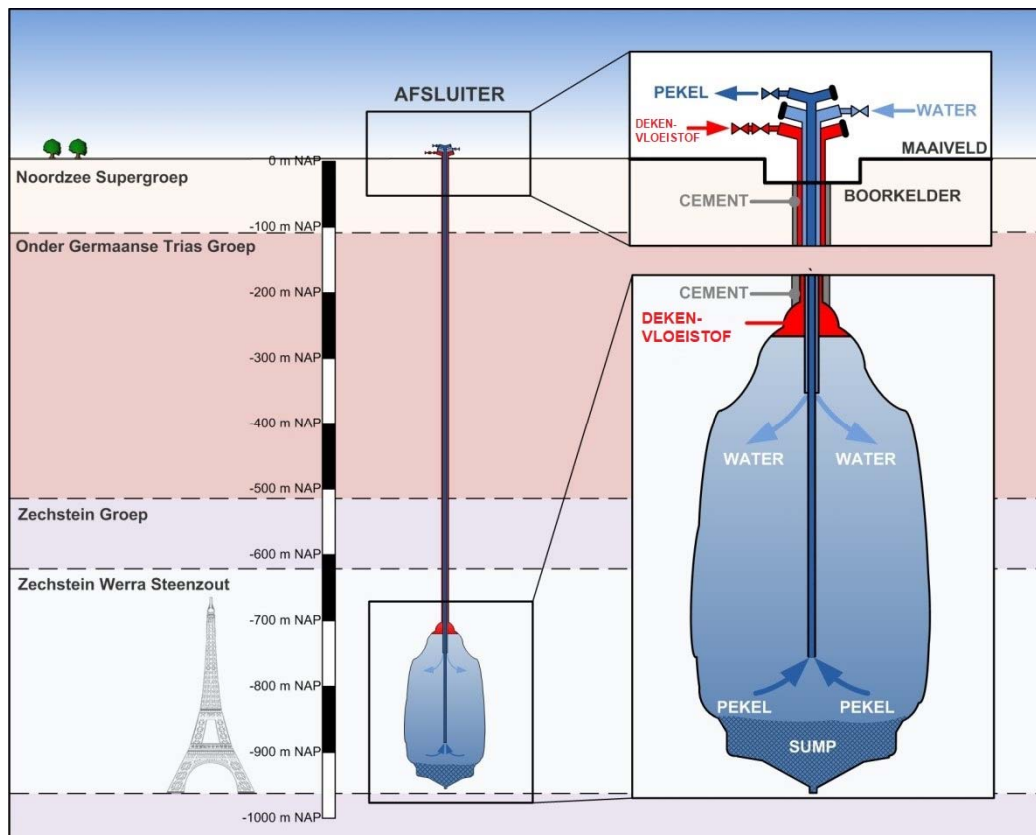
Figuur 3-5: Doorsnede van het uitlogingsproces van een caverne
