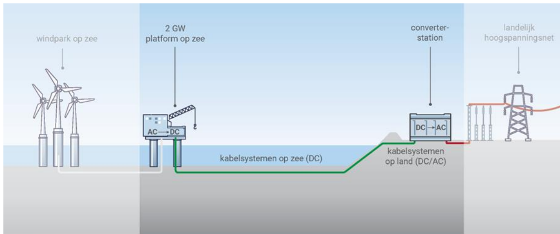
Afbeelding 2.1 Schematische weergave van het elektriciteitsnet (boven: gelijkstroom, onder: wisselstroom)
