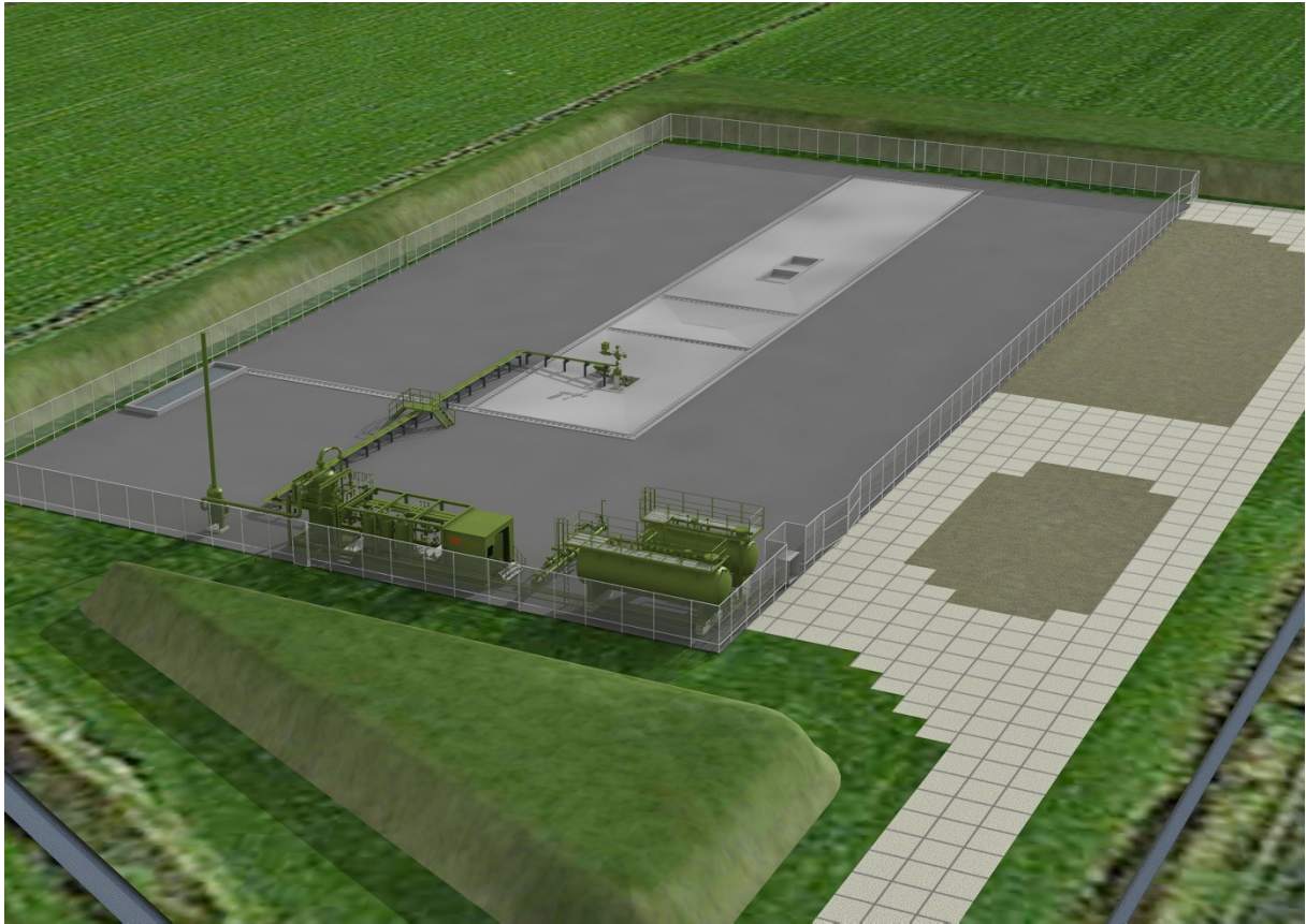
3D-view locatie Rottum vanuit het oosten
