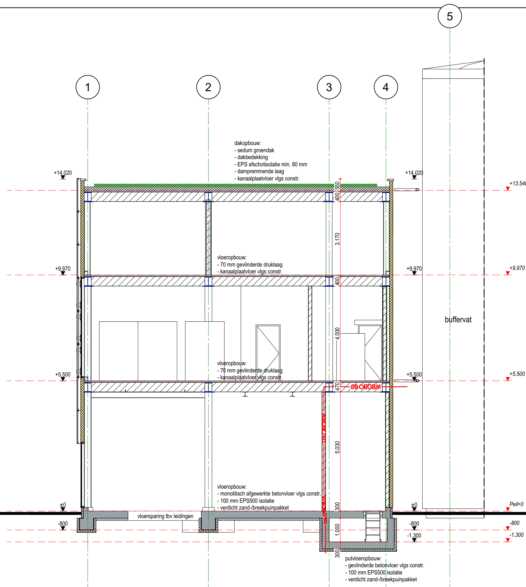
Doorsnede A-A FASE 1+2 - 1:100
