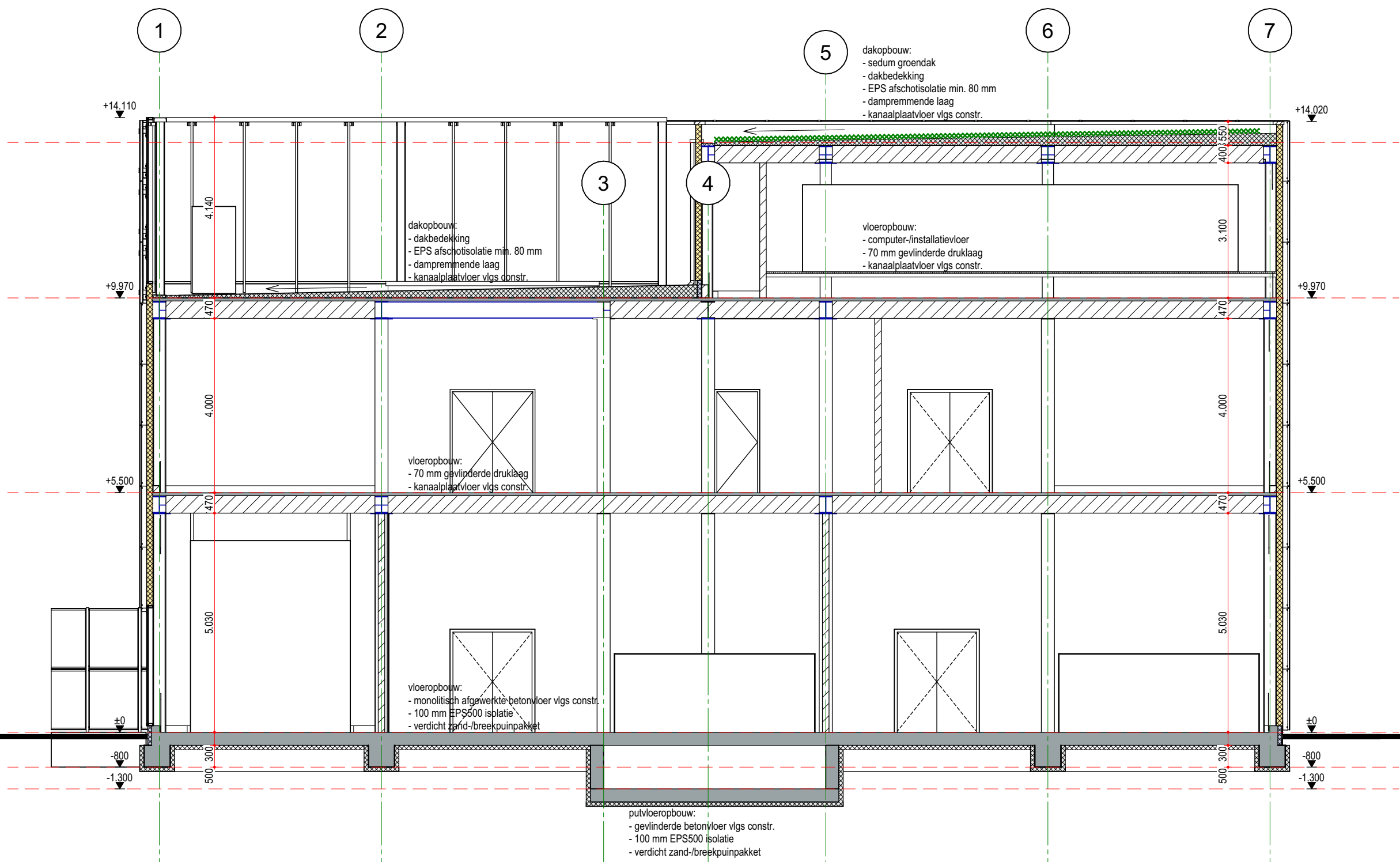
Doorsnede C-C FASE 1+2 - 1:100
