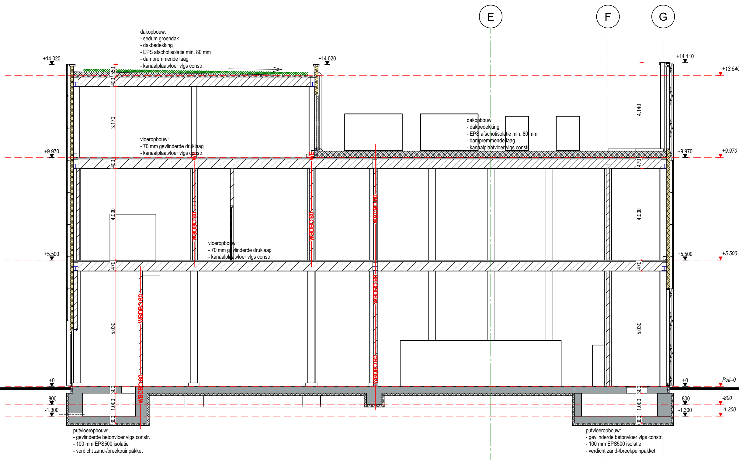
Doorsnede B2 FASE 1+2 - 1:100
