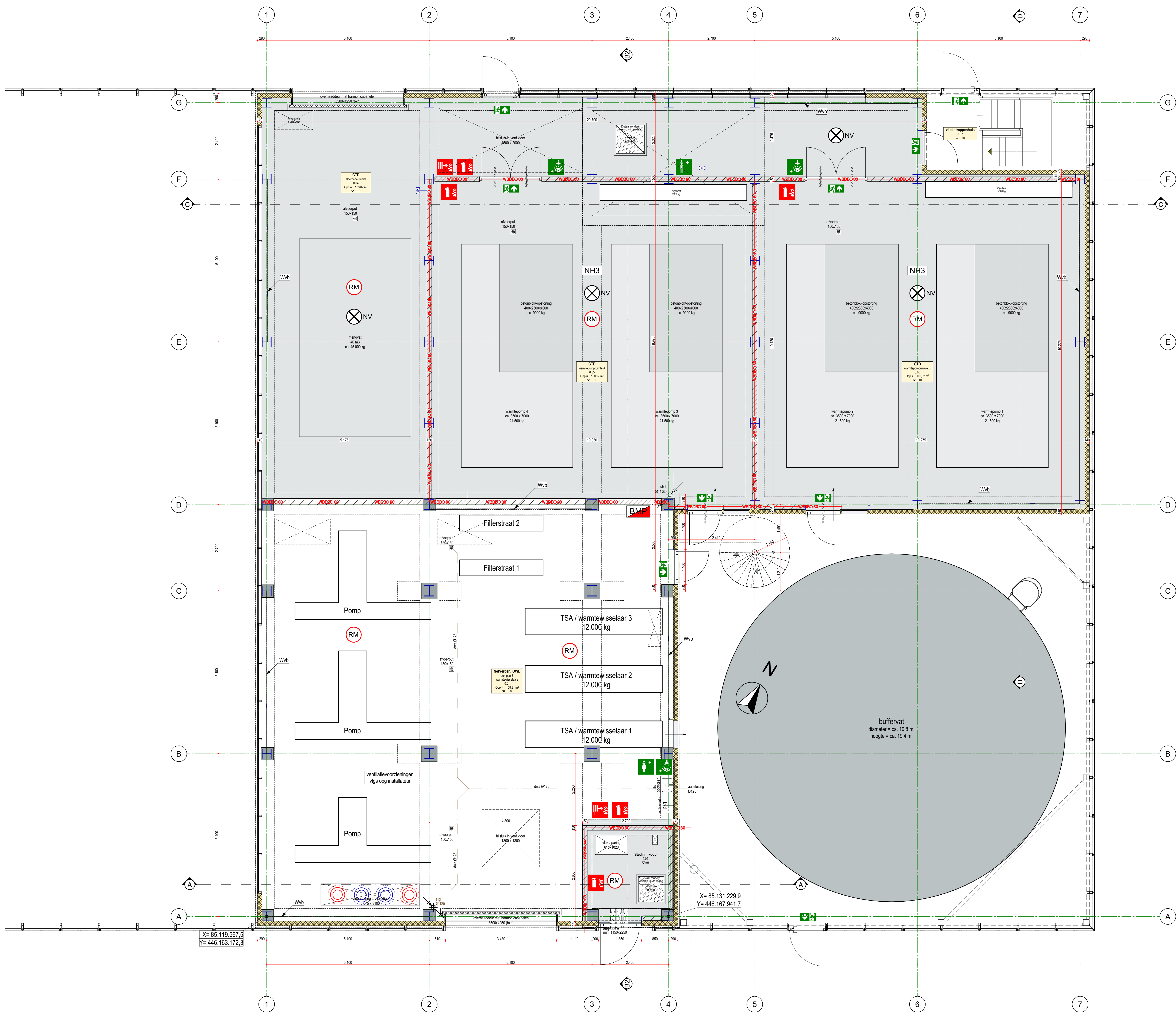
Begane grond 000+ FASE 1+2 - 1:50
