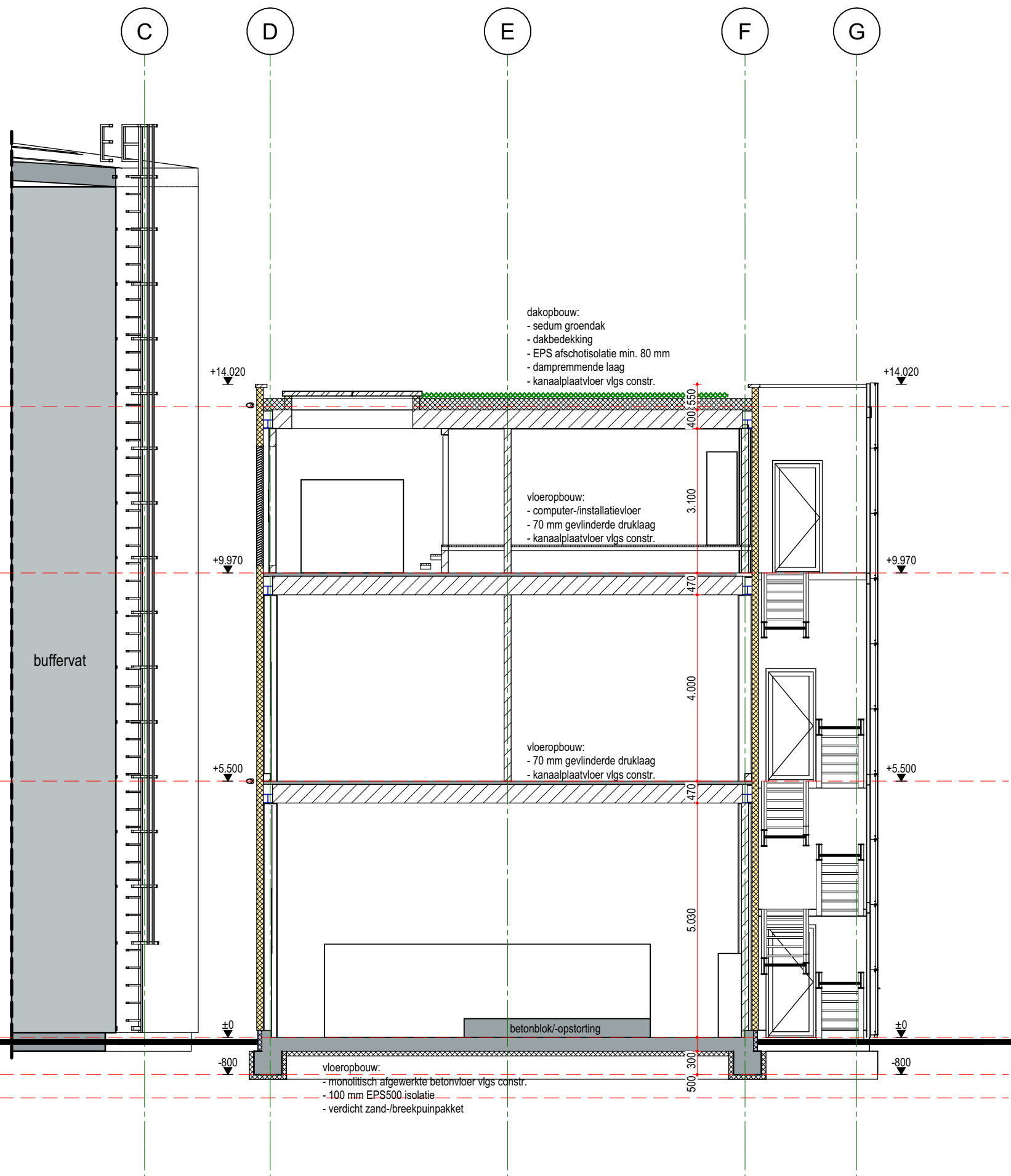
Doorsnede D-D FASE 1+2 - 1:100
