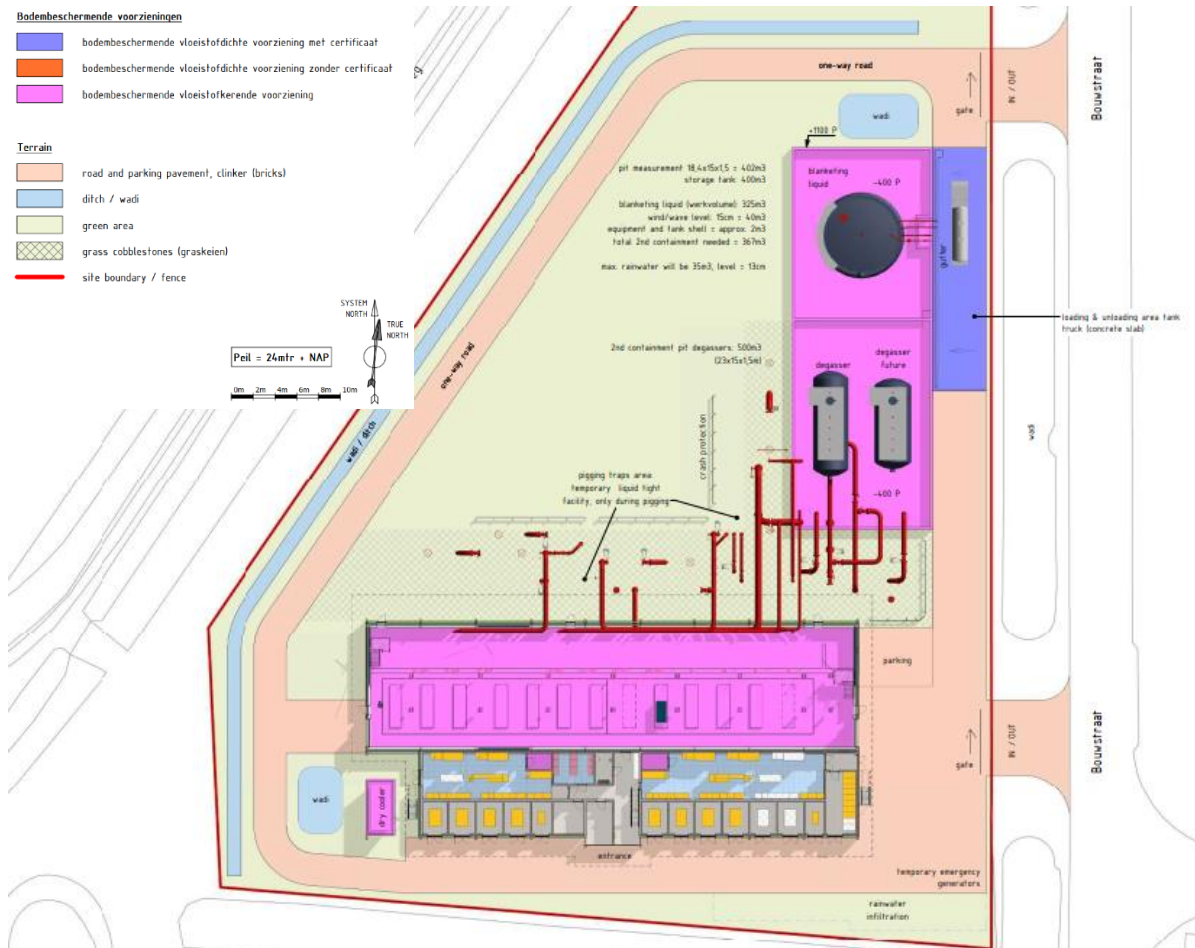
Figuur 2: Overzicht pompstation Stepelerveld
