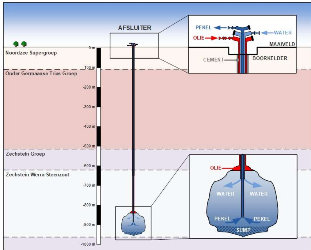
Figuur 6. Schematische weergave zoutwinningsproces in de ondergrond
