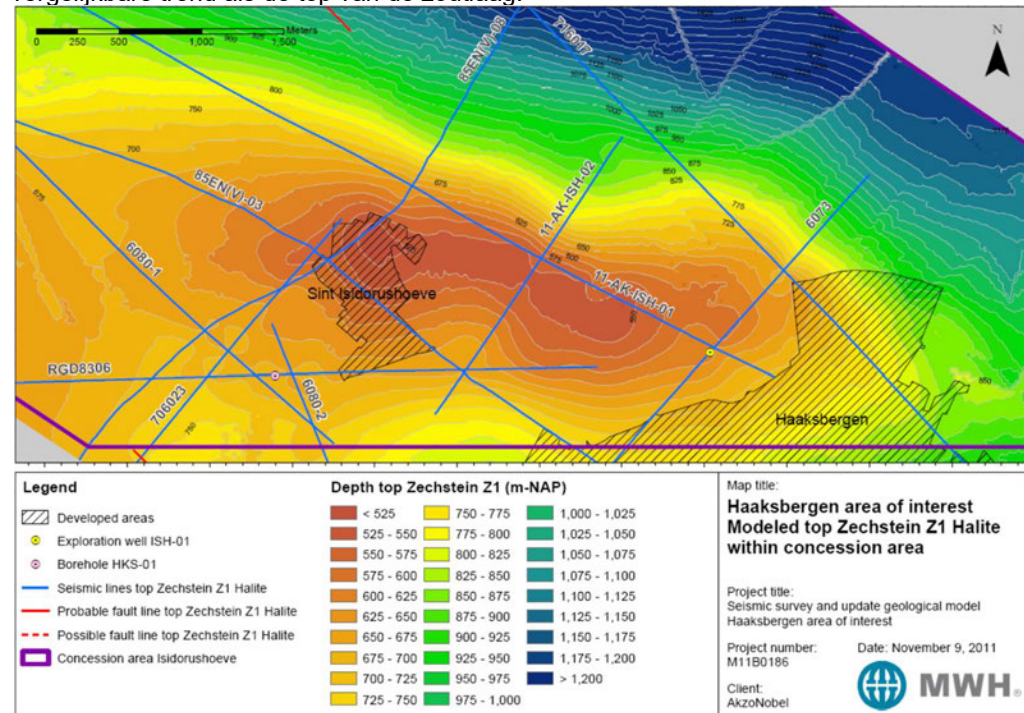
Figuur 2. Diepte top-zout in het Haaksbergen zoutvoorkomen
