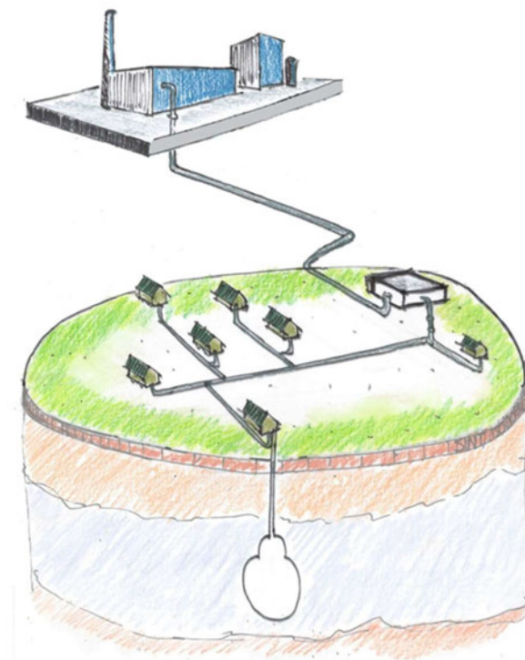
Figuur 5. Schematische weergave zoutwinning van caverne tot fabriek (niet op schaal)
