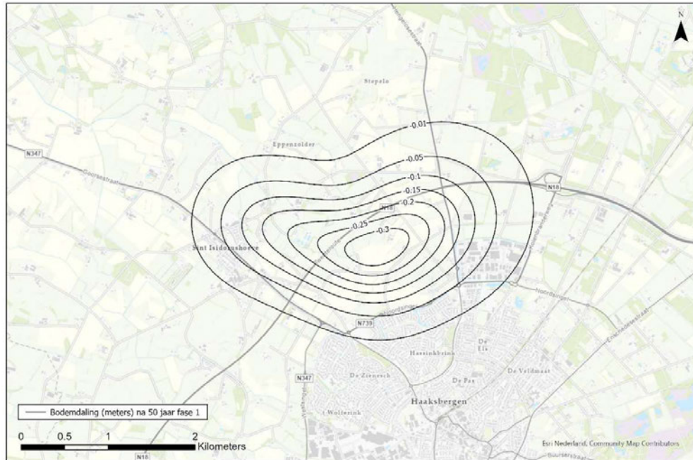
Figuur 13.: Bodemdalingsprognose in meters || 12 cavernes 50 jaar na aanvang productie || Scenario 2B (in het uiterste geval)
