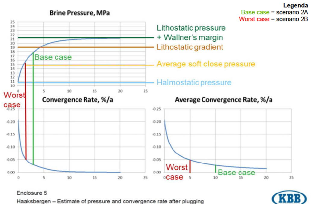
Figuur 14. Afnemende convergentiesnelheid en corresponderende drukken op basis van caveerne H-02 uit KBB 2012 met daaruit afgeleide constante convergentiesnelheden na sluiting voor de base case (scenario 2A) en worst case (scenario 2B) bodemdalingsscenario's.
