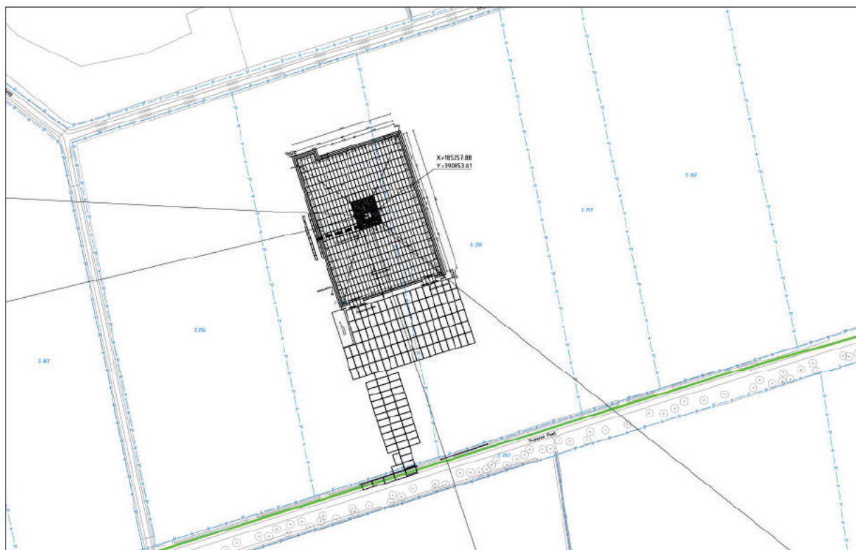
Figuur 3.1. Ontwerpplan boorlocatie met toegang vanuit het zuiden.
