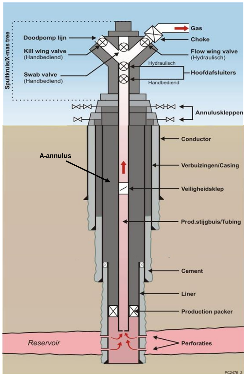
Figuur 3-1: Schematische weergave van een generieke gasproductie-put. De tekening is niet op schaal (sterk verticaal gekrompen)
