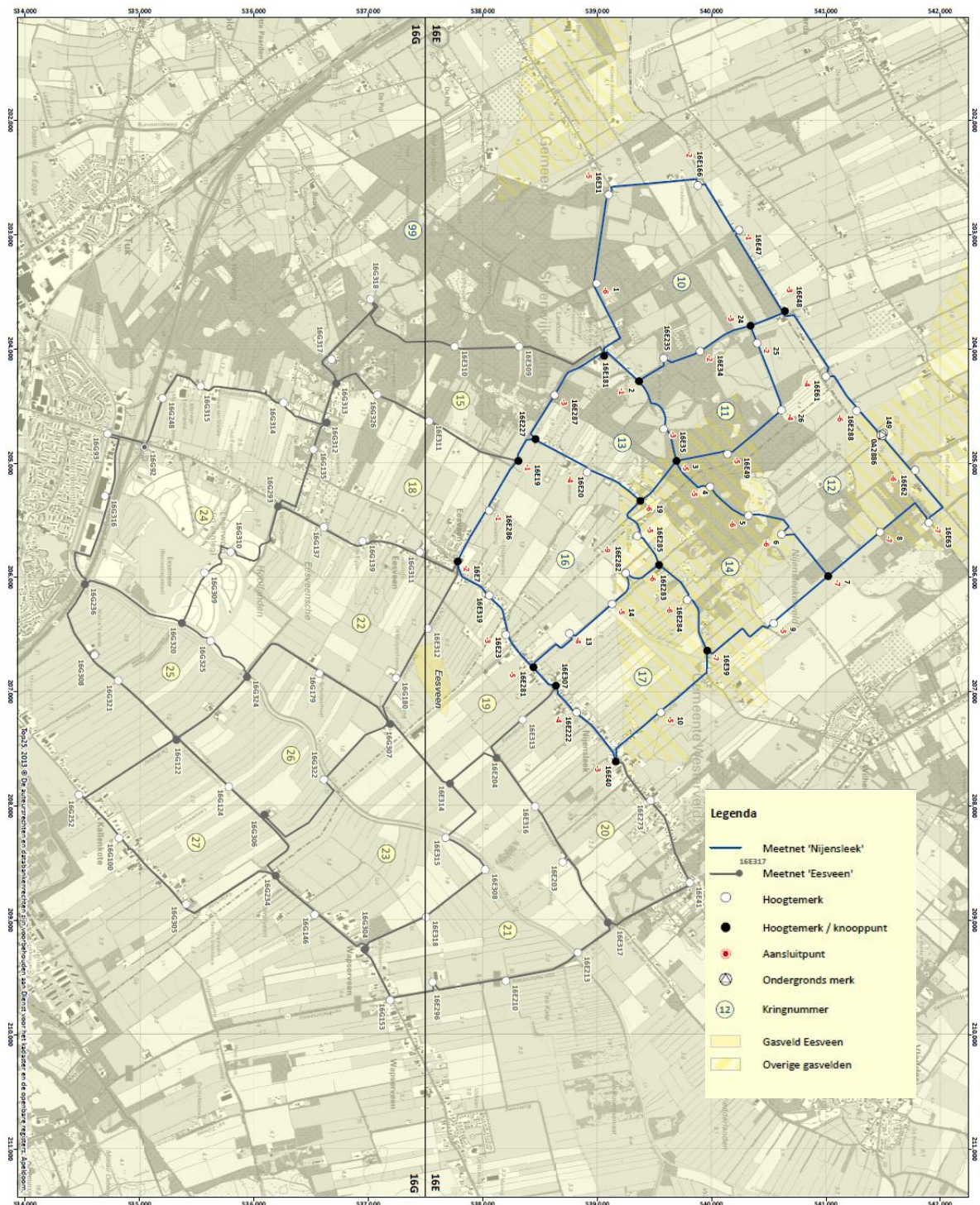
Figuur 16-1: Overzicht meetplan Nijensleek-Eesveen. De uitbreiding in 2015 naar Eesveen (ten SW van Nijensleek) is ook op de kaart weergegeven (zie ref. 14). Een verdere uitbreiding t.b.v. Eesveen-02 is in ontwerp.
