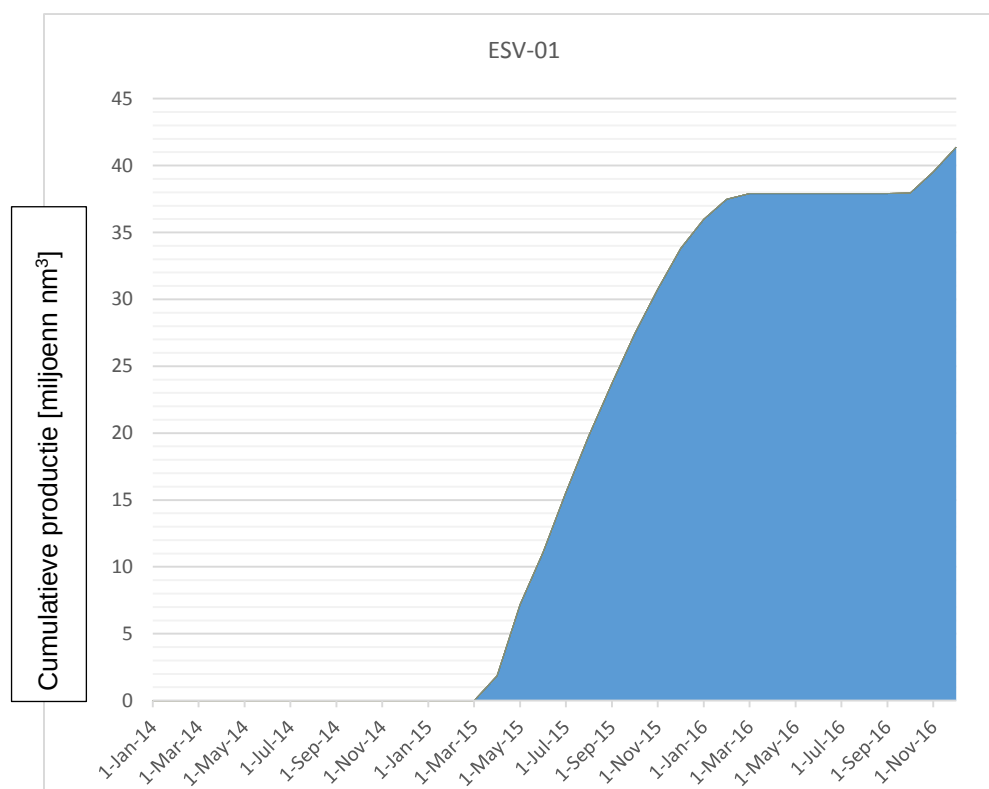
Figuur 5-2: Cumulatieve gasproductie historie Eesveen gasveld.
