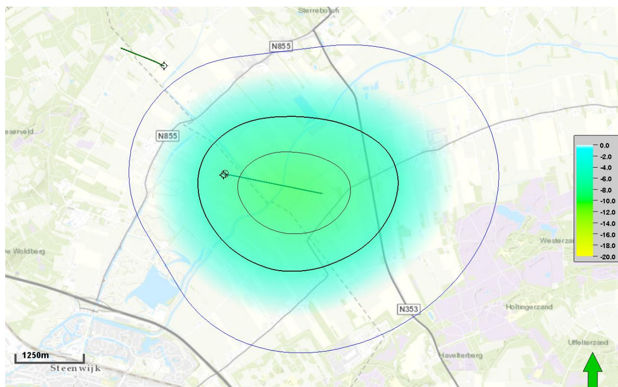
Figuur 6-6 Bodemdalingskom (P10) t.g.v. Eesveen winning. De blauwe lijn geeft het invloedsgebied, de kleuren de daling. Schaal is in mm. Contouren zijn 5, 8 mm. De geschetste situatie is die aan het eind van de winning. (Een uitvergroete versie is in de bijlage opgenomen.)
