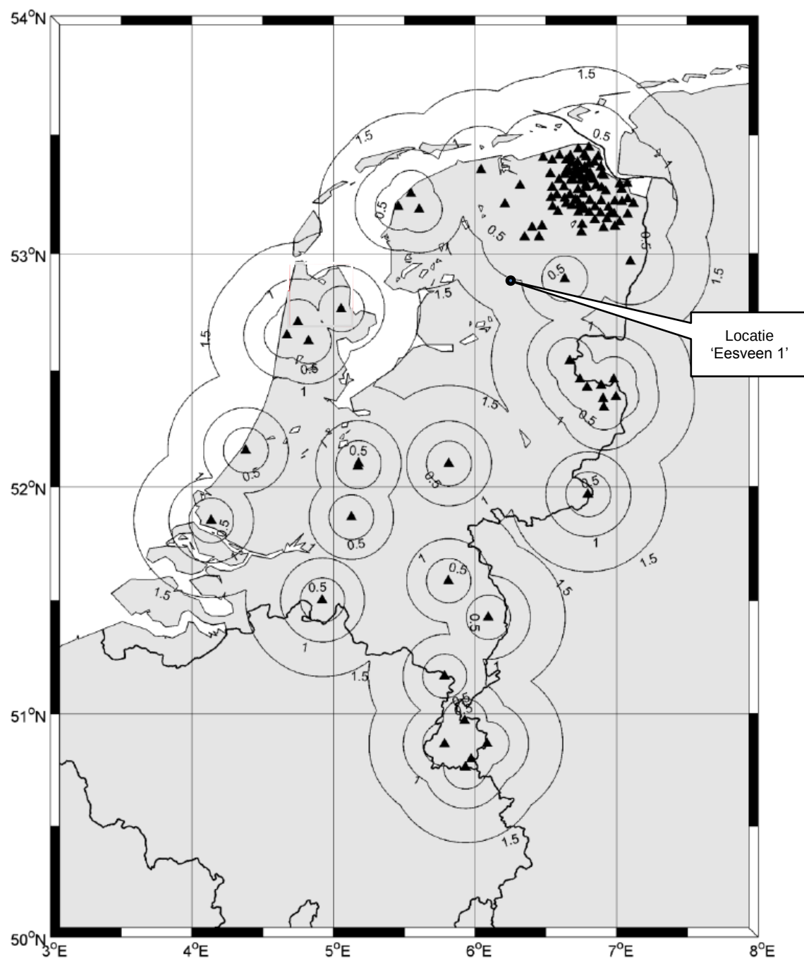
Figuur 17-4 Seismische detectie-stations en detectie-drempel-magnitude. Aangepast (met stations na 2010) naar Fig. 2a uit KNMI Ref. 10.
