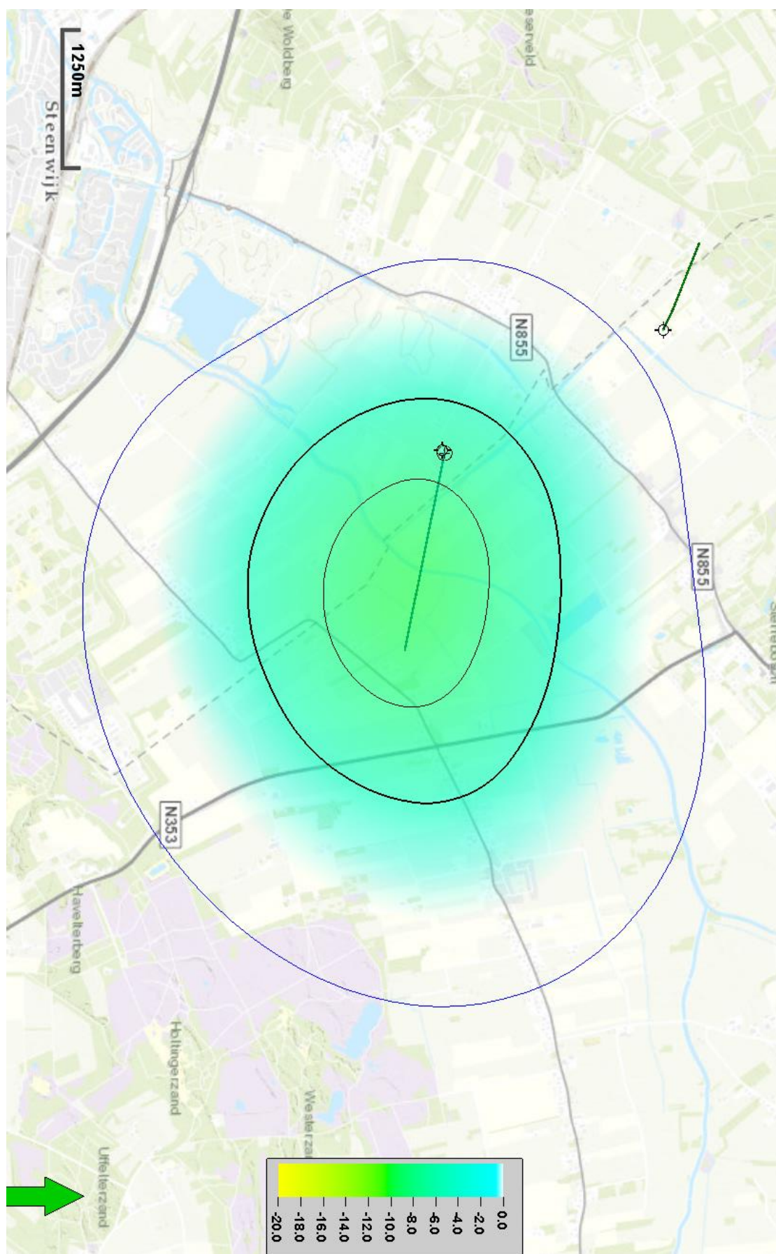
Figuur 15-1 Uitvergroting van Figuur 6-6, zie daar voor legenda [schaal in mm].
