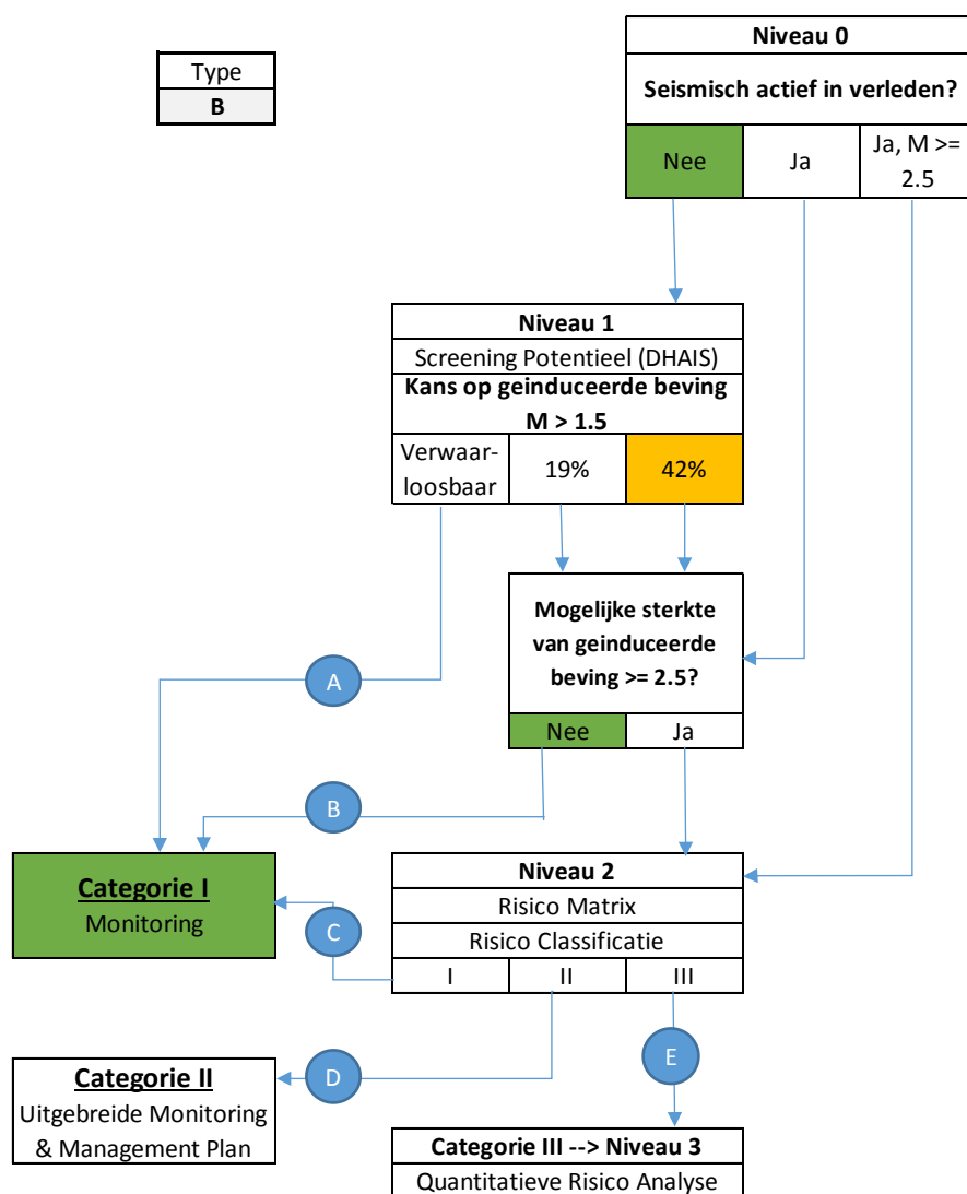
Figuur 17-1 SRA beslisboom toegepast voor Eesveen. De uitkomst is Categorie-I.
