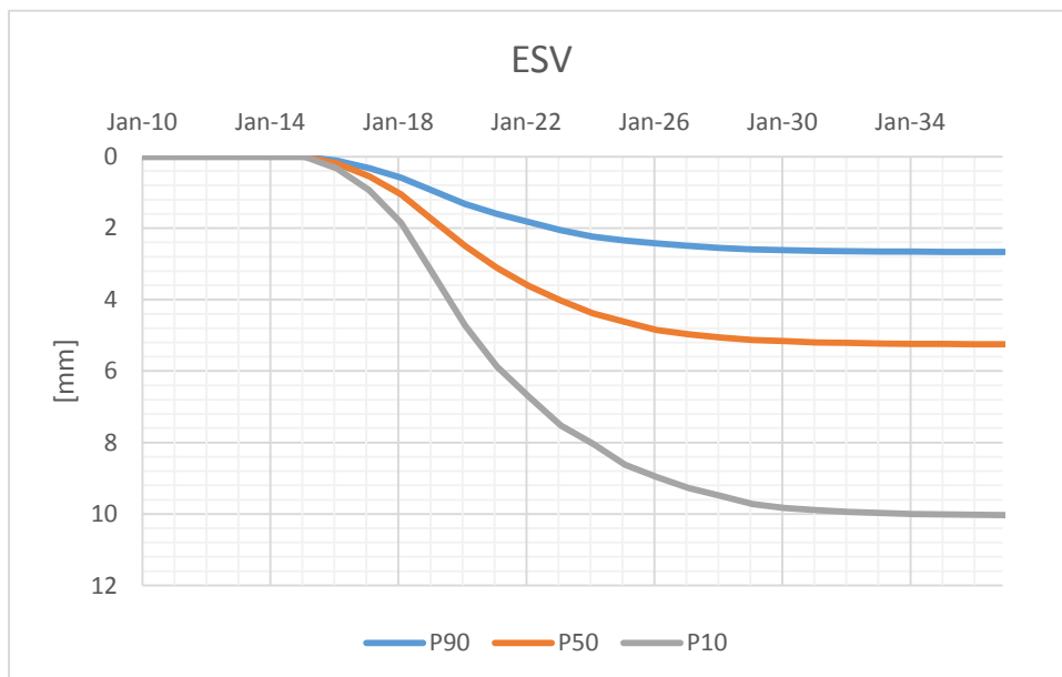
Figuur 6-5 Onzekerheid in het tijdsverloop van de Eesveen bodemdaling. P10 betekent hier een waarde waar de werkelijkheid met 90% zekerheid onderblijft (Figuur 6-5).
