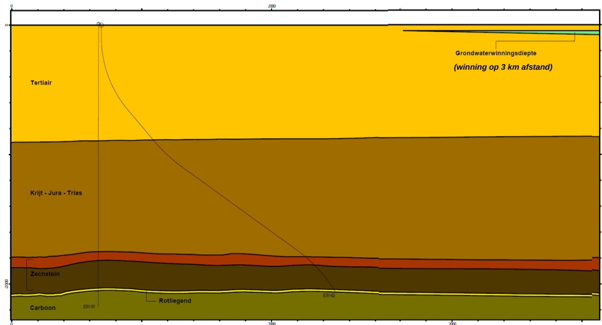
Figuur 4-2 Schematische weergave van de lagen boven het Eesveen voorkomen (ruwweg west → oost). De figuur is op schaal, i.e. niet verticaal uitvergroot. De Rotliegend, die hier vertegenwoordigd wordt door de Slochteren, waarin het gas zich bevindt, is de dunne gele strook tussen Carboon en Zechstein. De diepte waar winbaar grondwater zou kunnen zitten is geschetst. Daadwerkelijke winning vindt op 40-70m diep plaats, op 3 km van 'Eesveen 1'. [Schaal in m]
