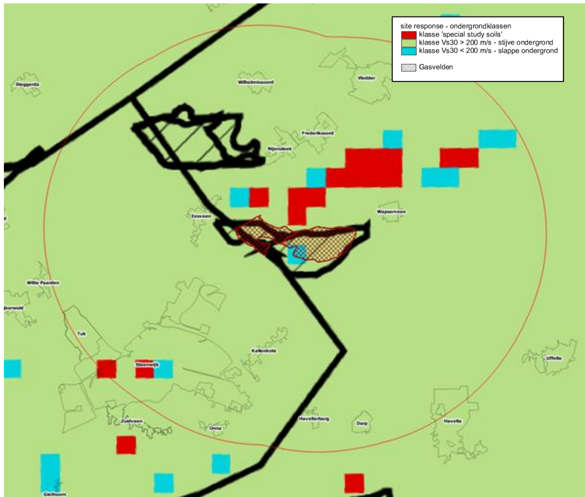
Figure 17-3 Grondsoorten in de buurt van het Eesveen voorkomen, gecategoriseerd naar mogelijke opslingeringseffecten (ref. 3). De rode cirkel geeft de 5 km straal in die relevant is voor de SRA. De zwarte contouren zijn zoals in de referentie (het weergegeven veld ten noordwesten is Nijensleek). Het doel van het kaartje is een inschatting van de fractie aan opslingeringsgevoelige grondopbouw, niet een locatie-specifieke detail-analyse (ref. 5).
