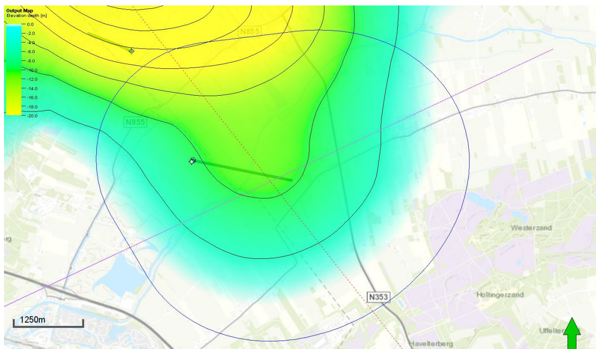
Figuur 6-8 Overlap van de oude Nijensleek dalingskom met de verwachte dalingskom voor Eesveen. Op het diepste punt van de Eesveen kom was enkele mm daling voordat de Eesveen winning begon. (vgl. Figuur 6-6). Schaal in mm, contouren 5, 8, 11, 14, 17 mm. De geschetste situatie is die aan het eind van de winning. De paarse & rode lijnen geven de secties aan waarlangs Figuur 6-7 is gemaakt.
