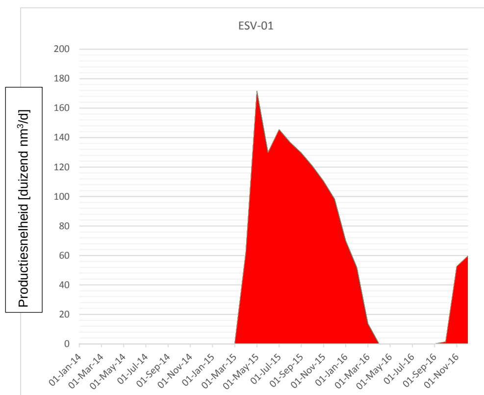
Figuur 5-1: Productie-snelheid historie Eesveen gasveld.
