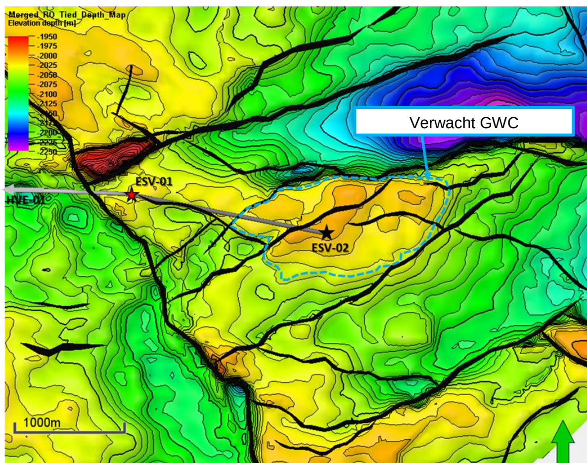
Figuur 14-1 Kaart van het ESV voorkomen, met de ESV-01 put, en de geplande gedeveerde ESV-02 put. Het pad van Havelte-01 put (HVE-01) is links-midden te zien. Het verwachte gas-water-contact (GWC) dat de uitgebreidheid van het voorkomen aangeeft, is weergegeven.
