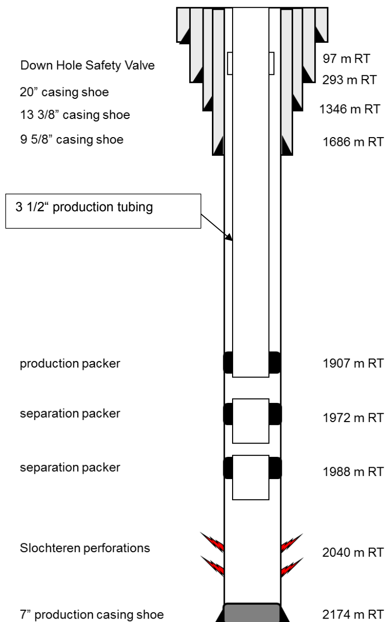
Figuur 3-2 Schematische weergave putverbuizing en -completie van de ESV-01 put. De tekening is niet op schaal (sterk verticaal gekrompen).
