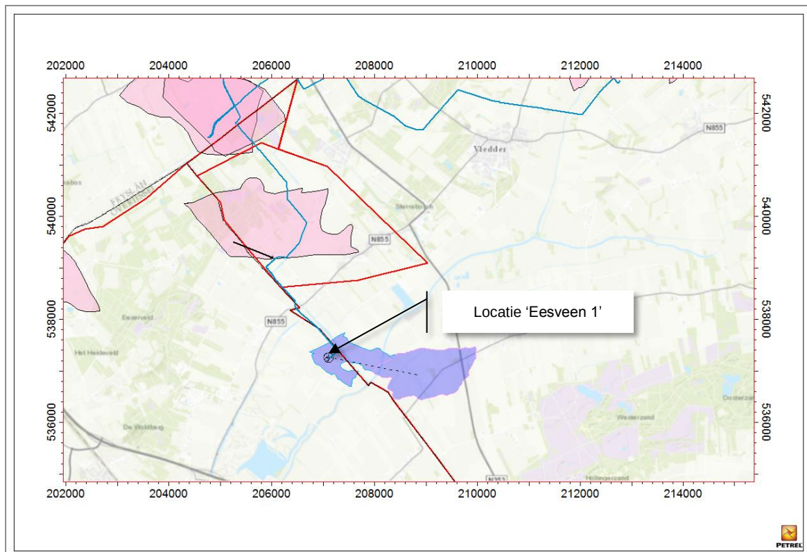
Figuur 2-2: Topografische kaart Eesveen gas veld met putten en pijpleidingen (blauw). De locatie 'Eesveen 1' is met een pijl aangeduid. De geplande ESV-02 put is gestippeld. De bestaande ESV-01 put is verticaal. Concessiegrenzen in rood. De roze vlakken geven nabijgelegen velden aan. Meteen ten noordwesten ligt het uitgeproduceerde voorkomen Nijensleek, nu in gebruik als water-injectie locatie.
