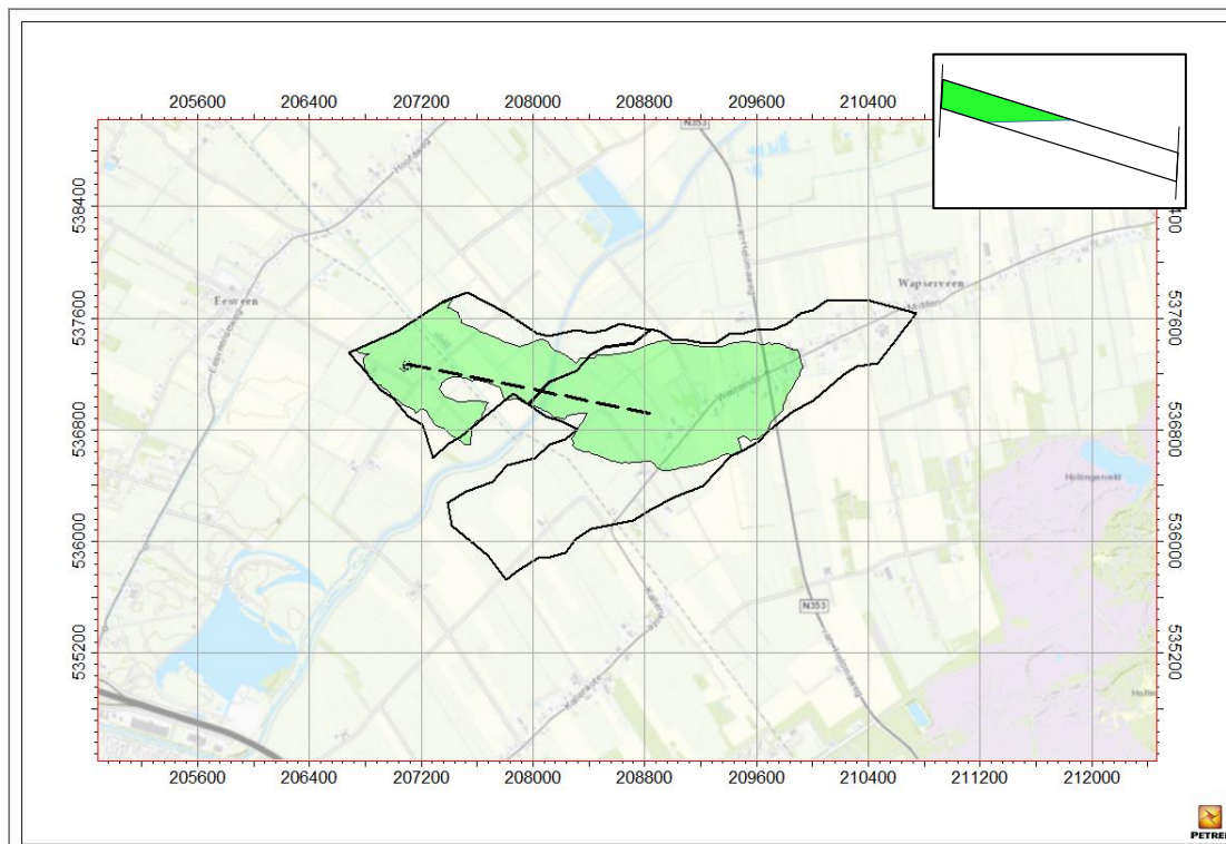
Figuur 6-3: Meenemen van het watervoerende deel in de bodemdaling berekening. De inzet rechtsboven geeft de methode (groen is gas, wit is water in breukblok), de kaart geeft de uitwerking voor Eesveen. Merk op dat het gedrag van ESV-01 consistent is met een afwezig drukeffect van het water (paragraaf 5.2).
