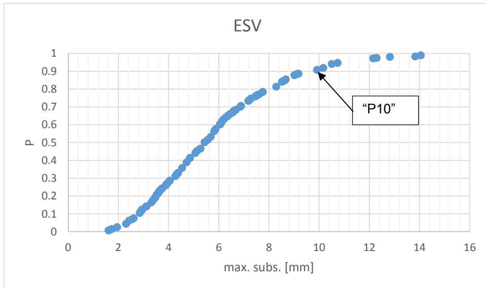
Figuur 6-4 Cumulatieve kansverdeling voor de uiteindelijke Eesveen bodemdaling. De daling blijft met 90% zekerheid onder de 10 mm. Die waarde wordt ook "P10" genoemd.
