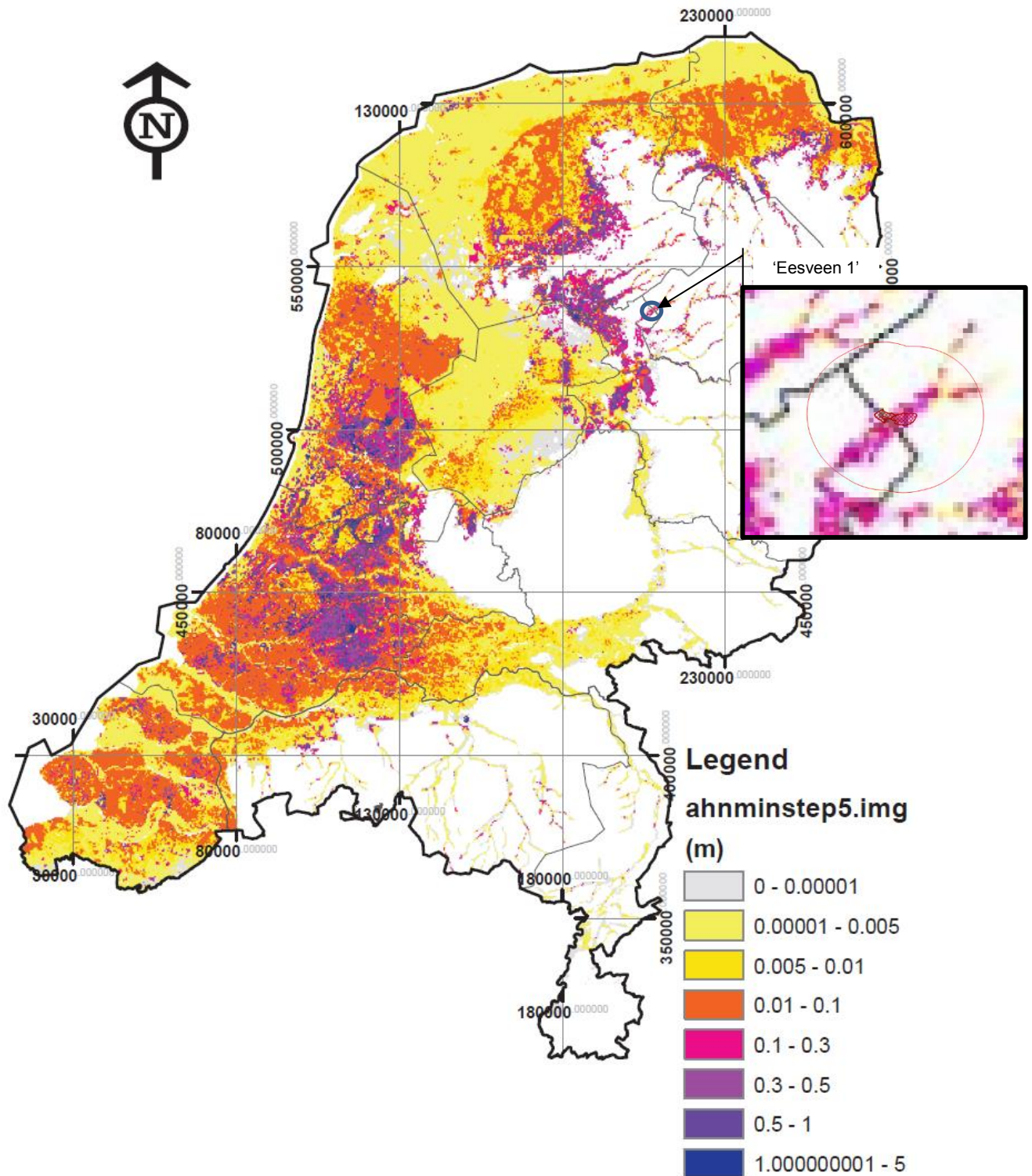
Figuur 6-2: Autonome bodemdaling 50 jaar na 2011 (Deltares, ref. 1), schaal in m. De locatie van Eesveen is aangegeven, de inzet geeft een uitvergroting. De rode cirkel geeft een straal van 5 km rond het voorkomen.
