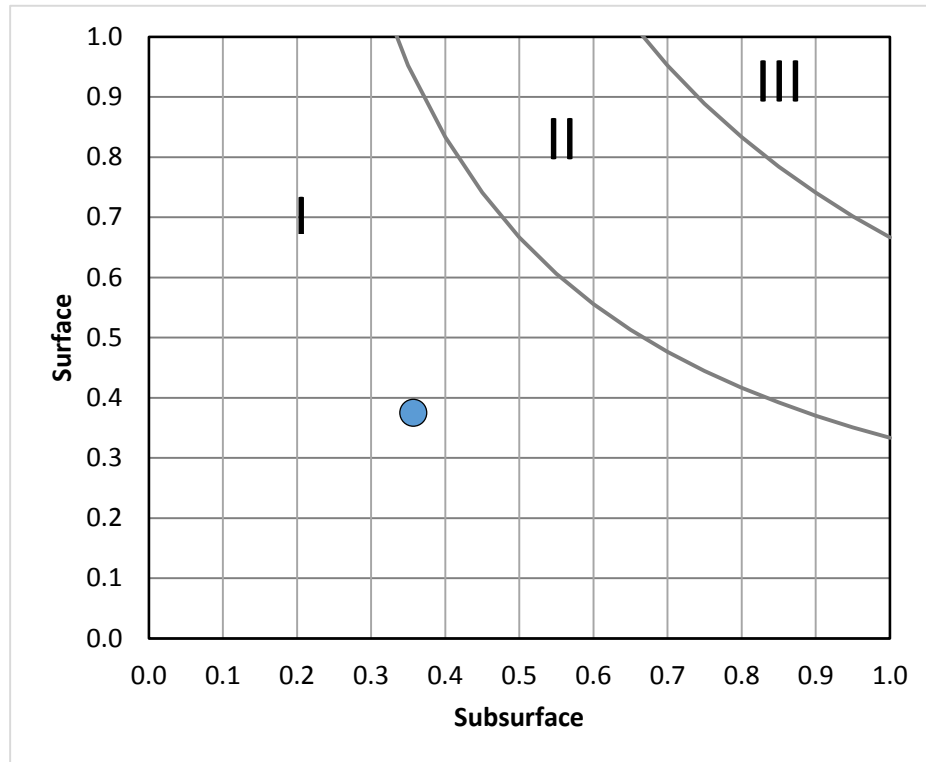
Figuur 17-2 Resultaat van een Niveau-2 analyse voor Eesveen. Deze analyse is niet verplicht (de maximaal realistische magnitude is onder de 2.5), maar de grafiek laat zien dat het resultaat ruim in categorie I valt, zelfs al zouden we de analyse wel doen.
