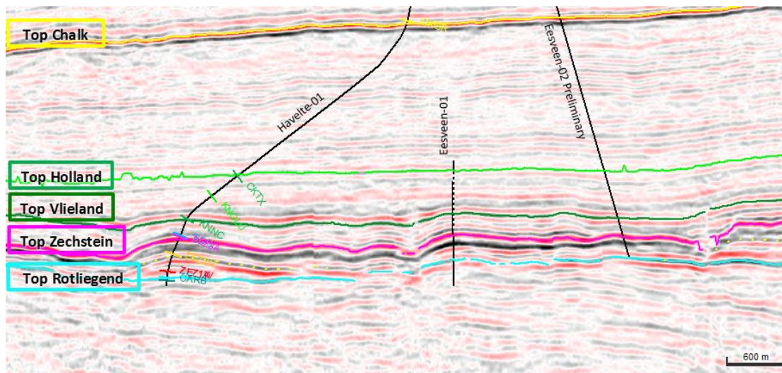
Figuur 4-1: Doorsnede van Eesveen Slochteren reservoir (ruwweg west→oost) met put projecties. De exploratieput Havelte-01 is ook weergegeven (metingen uit deze put zijn ook gebruikt). De verticale schaal geeft de tijd aan die seismische golven heen-en-weer onderweg zijn. Zie Figuur 4-2 voor een schematische interpretatie.
