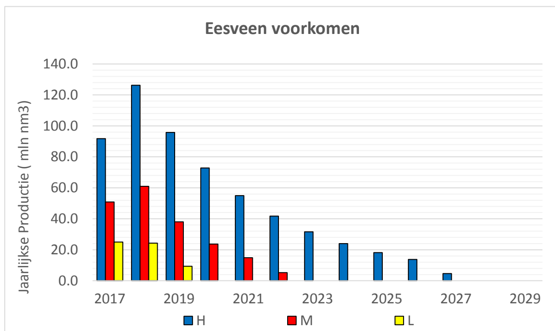
Figuur 5-3: Eesveen voorkomen productie voorspellingen. Zie tekst voor een beschrijving van de redenen voor onzekerheid in productie-hoeveelheid en -snelheid.
